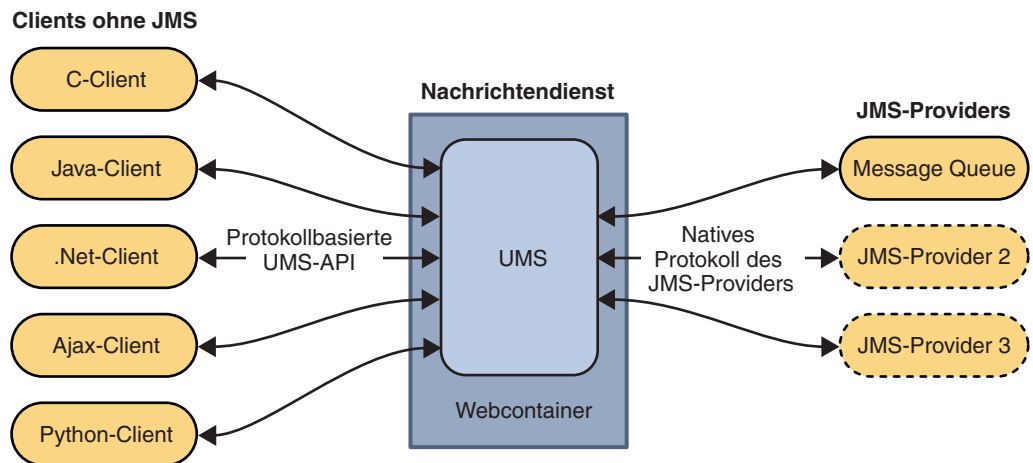
ABBILDUNG 1-1 UMS-Architektur
