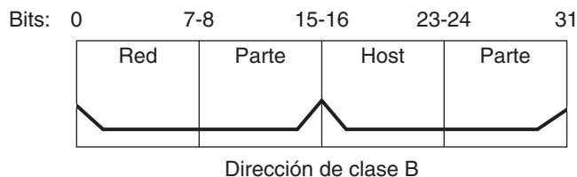
FIGURA 10-4 Asignación de bytes en una dirección de clase B
