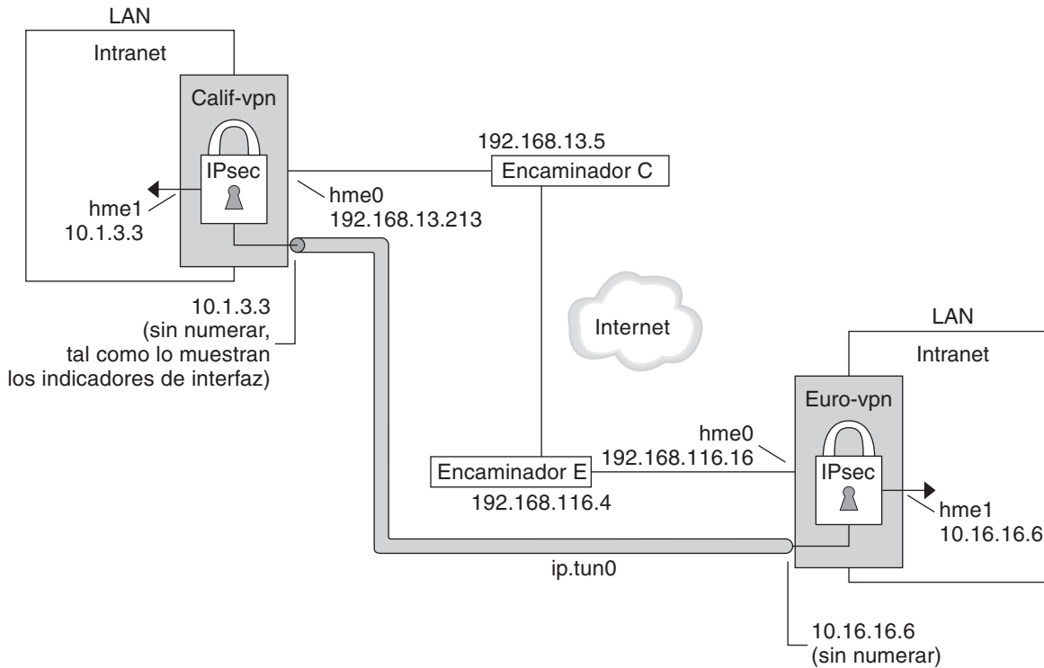
FIGURA 20-2 VPN de ejemplo entre oficinas separadas por Internet
