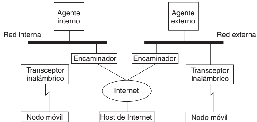
FIGURA 27-1 Topología de IP para móviles
