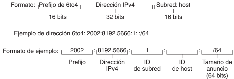
FIGURA 11-2 Partes de un prefijo de subred de 6to4
