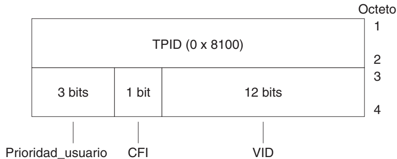
FIGURA 5-4 Formato de encabezado de etiqueta de Ethernet
