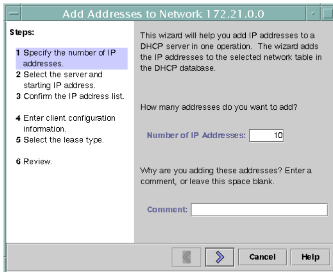
FIGURA 15-9 Asistente Add Addresses to Network del Administrador de DHCP
