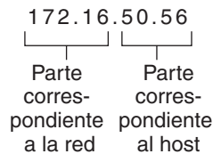
FIGURA 2-1 Formato de direcciones IPv4
