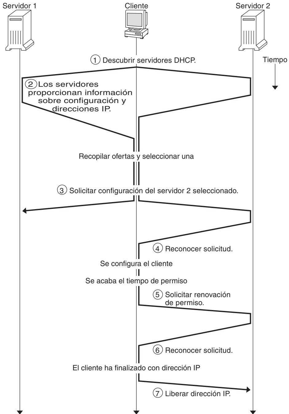
FIGURA 12-1 Secuencia de eventos para el servicio DHCP
