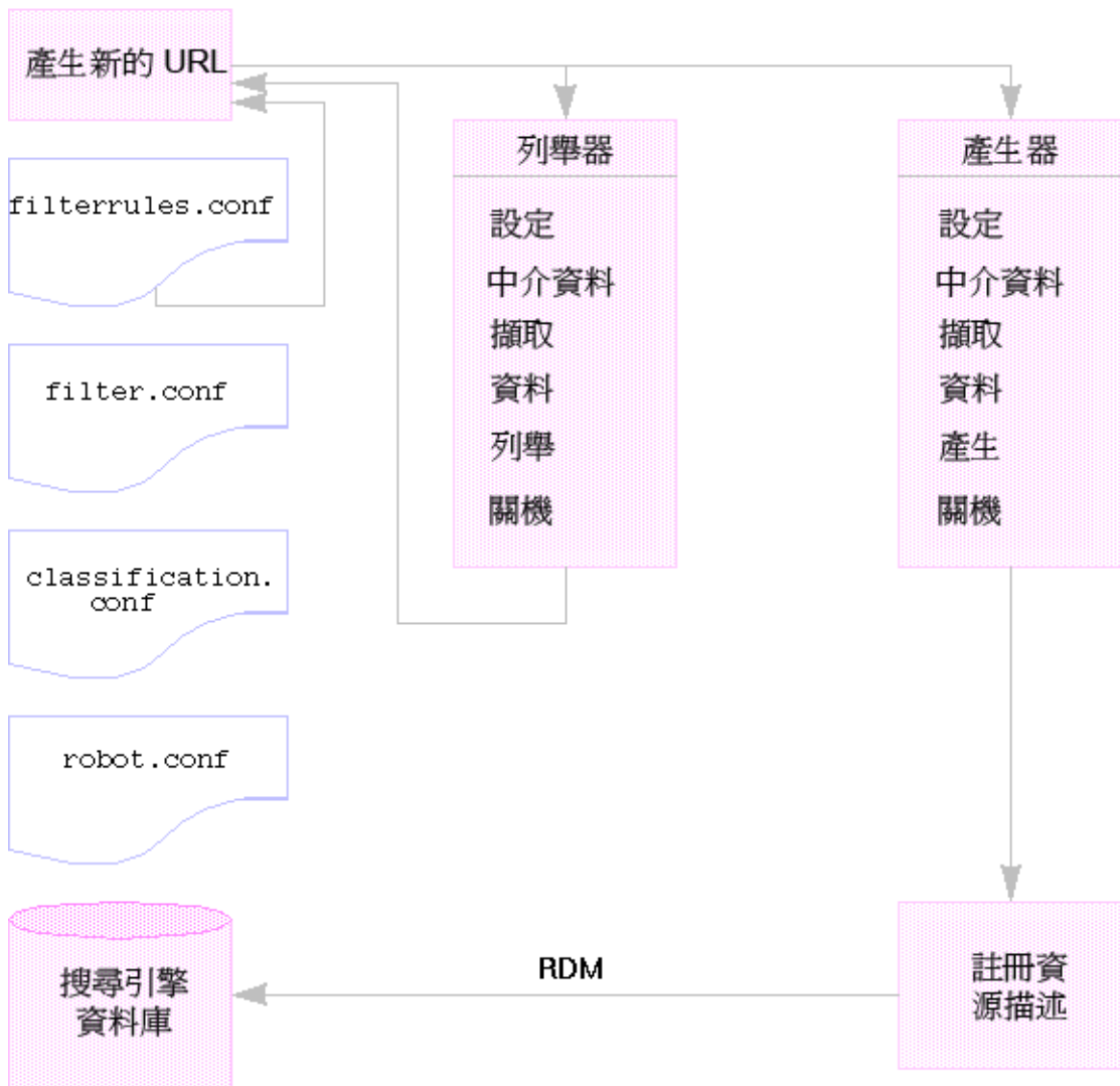
圖 19-1 網頁抓取程式的作業方式
