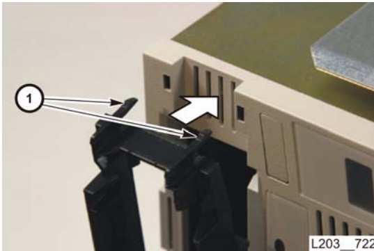
SDLT Drive Bezel
