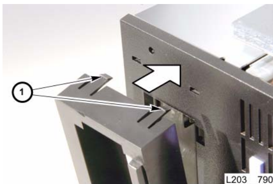
IBM Drive Bezel
