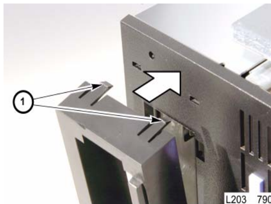
IBM Drive Bezel
