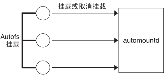
图 6-3 svc:/system/filesystem/autofs 服务启动 automount
