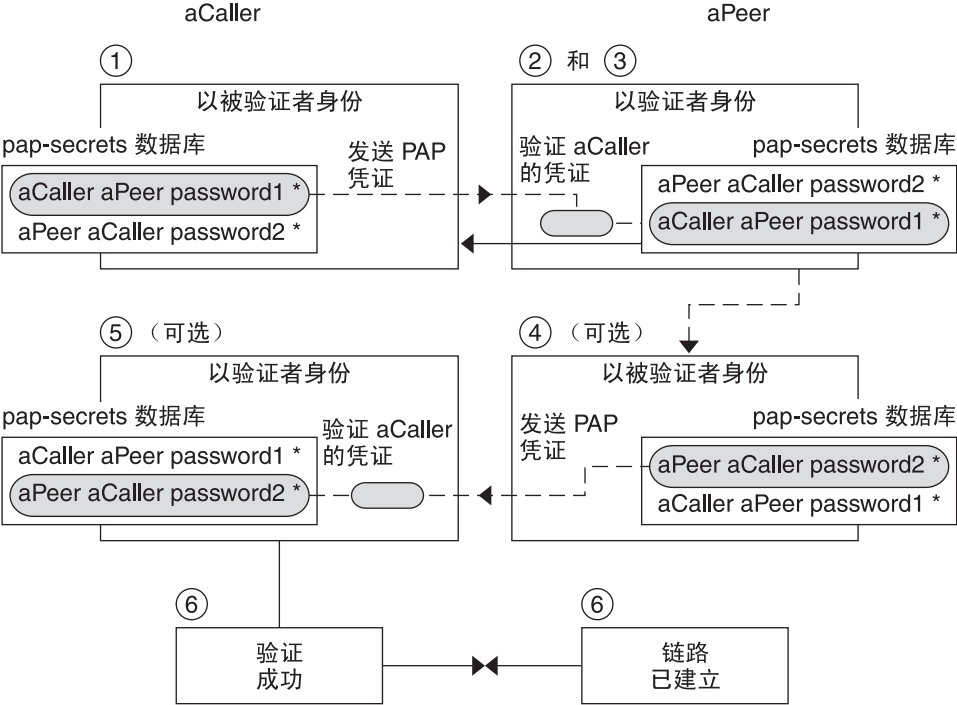
图 22-1 PAP 验证流程
