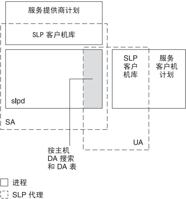
图 7-3 SLP 实现
