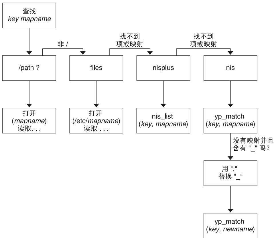
图 6-6 Autofs 使用名称服务的方式
