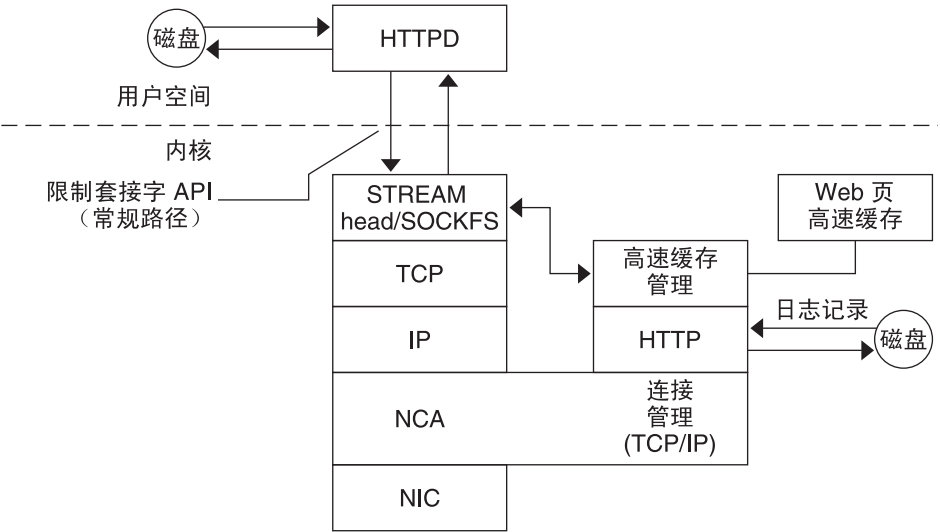
图 2-1 NCA服务的数据流
