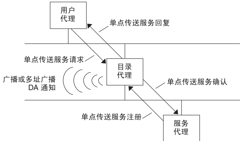
图 7-2 用 DA 实现的 SLP 体系结构代理和进程
