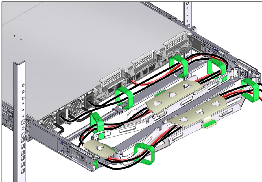
Figure 5.17. CMA avec câbles installés, capots de câbles fermés et câbles fixés avec bandes Velcro
