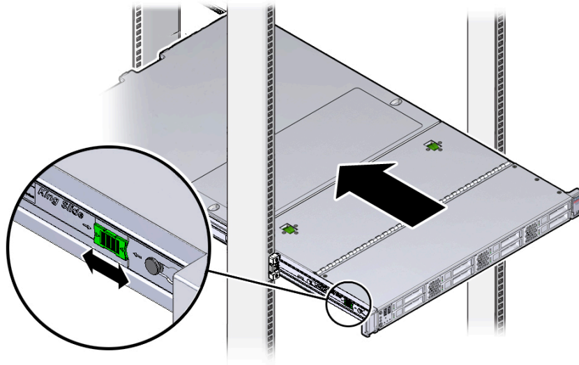
Figure 5.16. Emplacement des onglets de dégagement de la glissière
