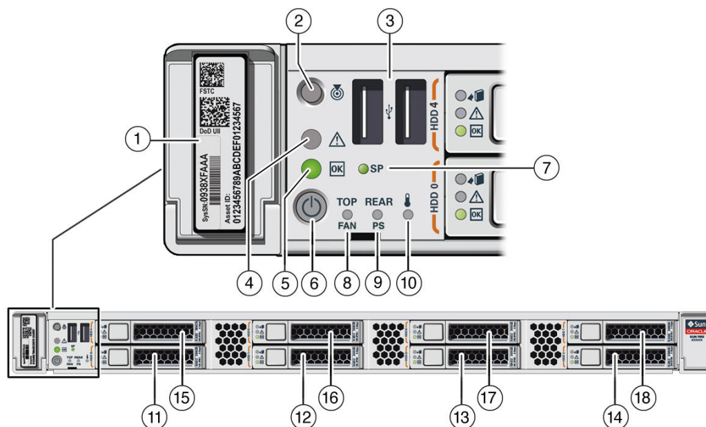
Figure 3.1. Configuration d'un panneau avant de serveur avec huit unités 2,5 pouces
