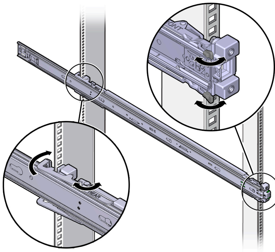
Figure 5.5. Alignement de l'ensemble glissière avec le rack
