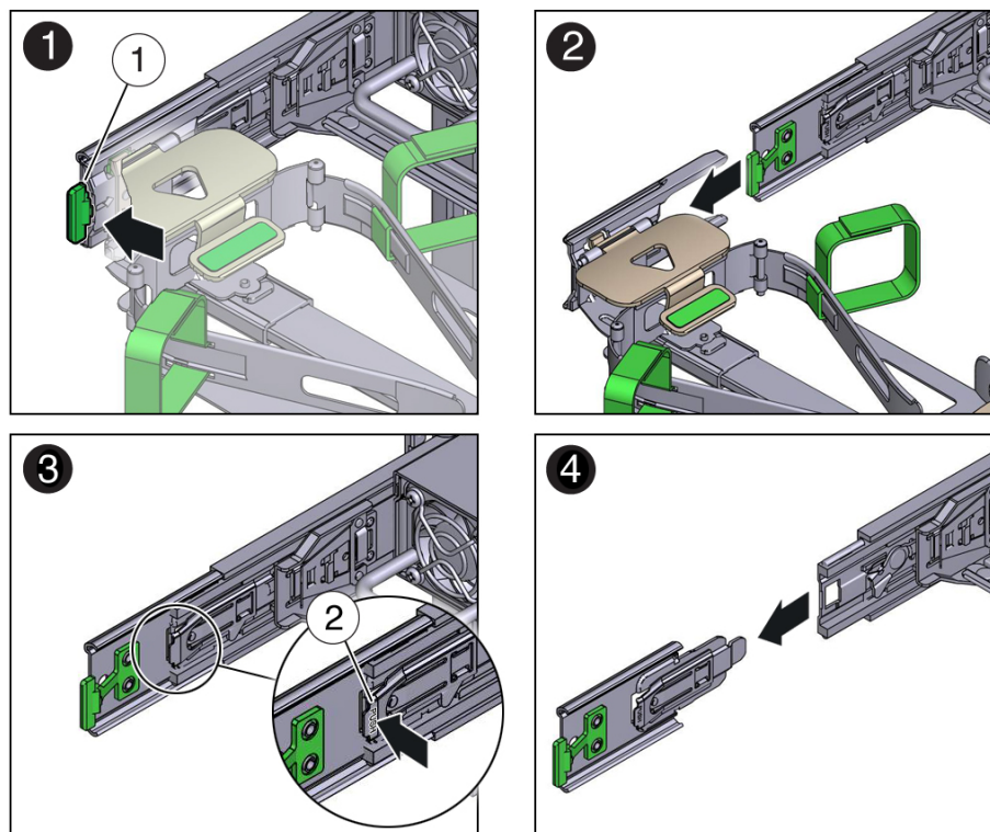
Figure 5.18. Déconnexion du connecteur D
