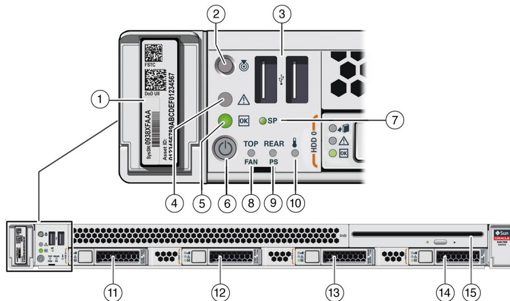
Figure 3.2. Configuration de panneau avant de serveur avec quatre unités 2,5 pouces et lecteur DVD SATA
