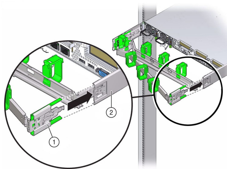
Figure 5.23. Insertion du connecteur de glissière du module de fixation des câbles dans la glissière droite
