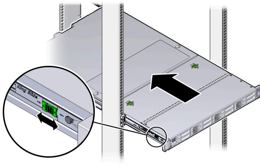
Figure 5.26. Emplacement des onglets de dégagement de la glissière
