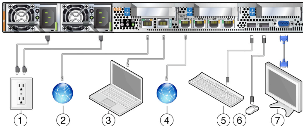
Figure 6.1. Référence de câblage du panneau arrière
