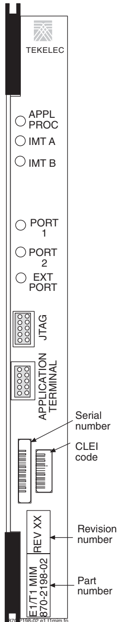
Figure A-7. E1/T1 MIM)
