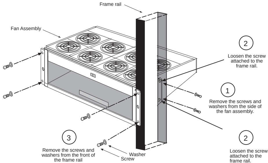
Figure A-24. Remove Fan Assembly
