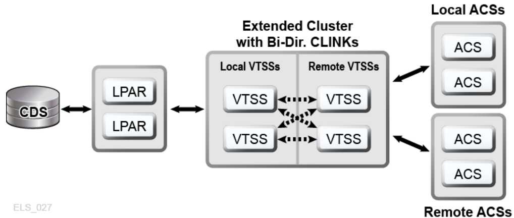
図1.7 D-HA 拡張クラスタ構成 (オフサイトのボールドを除く)
