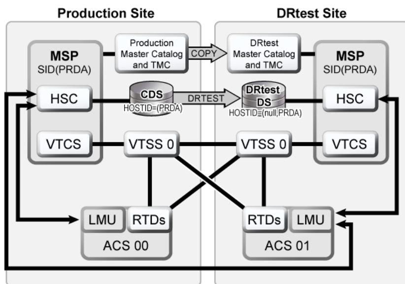
図6.2 スペア VTSS 構成 - DRTEST ユーティリティの実行後
