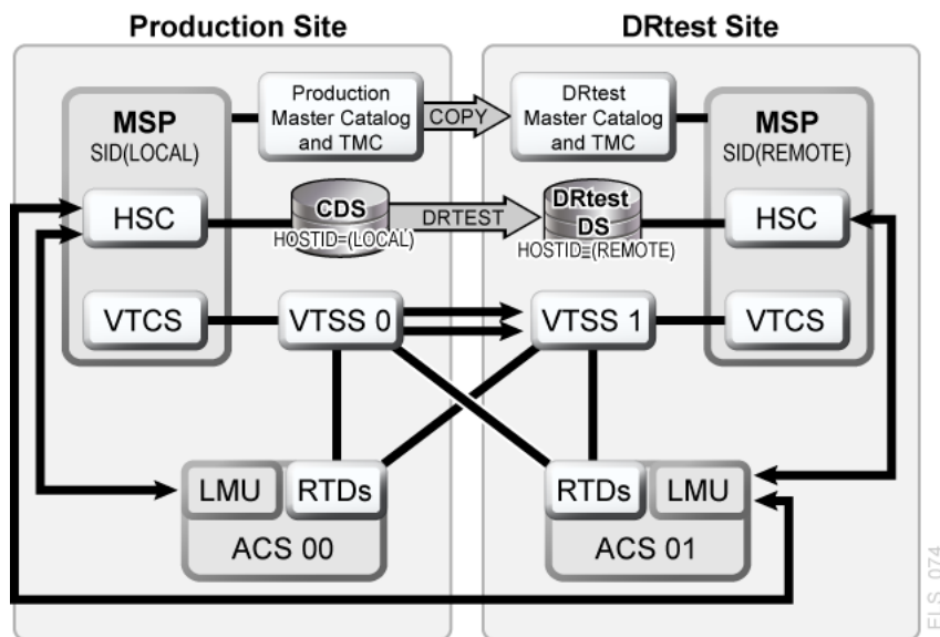
図6.8 プライマリ/セカンダリクラスタ VTSS の構成 - テスト中
