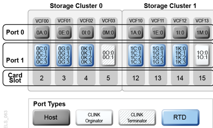
図A.5 VSMRP2 - 8 枚の VCF カード、8 つのホストポート、24 個の RTD 用の FICON ディレクタ、4 つの CLINK が搭載された VSM5
