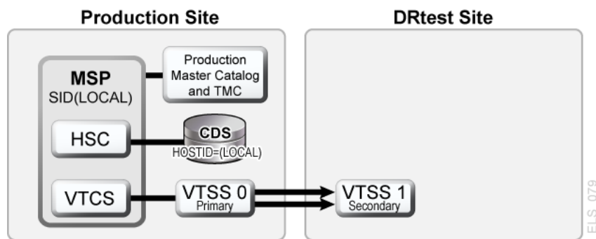
図6.13 プライマリ/セカンダリクラスタ VTSS テープレス構成 - DRTEST ユーティリティーの実行前
