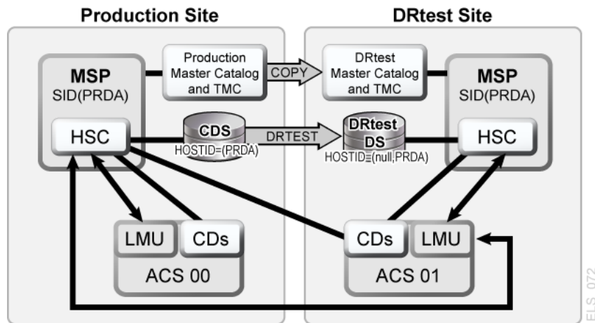
図6.6 読み取り専用構成 - DRTEST ユーティリティの実行後
