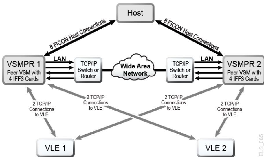
図A.8 VLE に相互接続された、TCP/IP CLINK による VSM5 と VSM6 間のクラスタ
