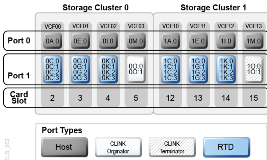
図A.4 VSMMPR1 - 8枚の VCF カード、8つのホストポート、24個の RTD 用の FICON ディレクタ、4つの CLINK が搭載された VSM5
