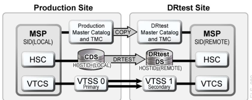
図6.14 プライマリ/セカンダリクラスタ VTSS テープレス構成 - テスト中
