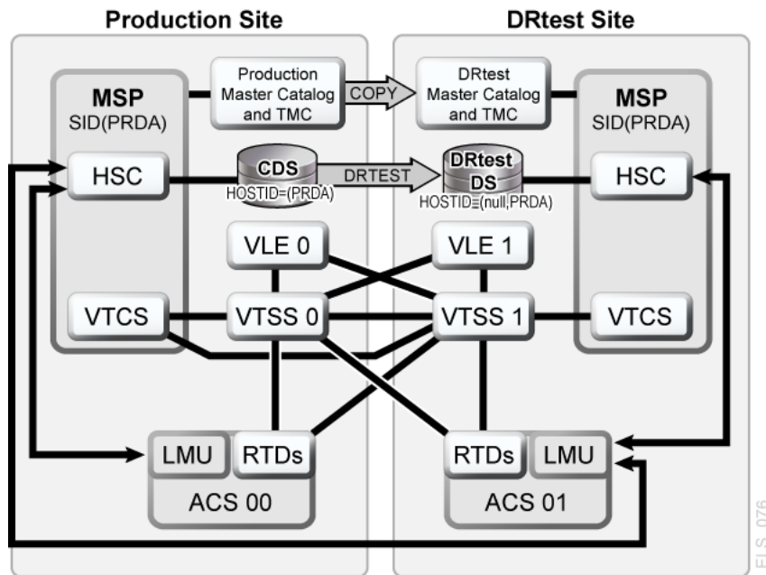
図6.10 VLE および ACS の構成 - DRTEST ユーティリティの実行後
