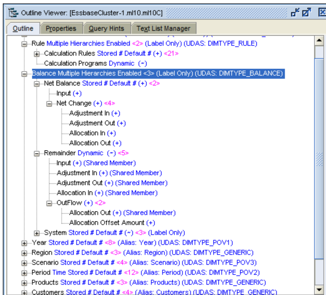
Figura 5-3 Esquema de la dimensión Balance de Management Ledger
