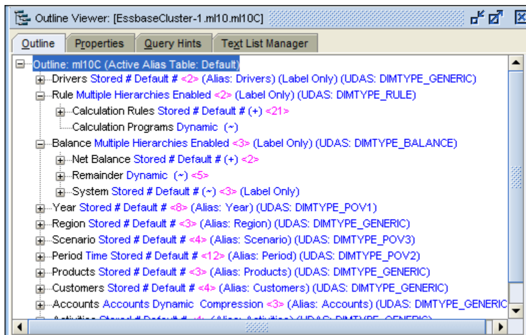
Figura 5-1 Esquema de Essbase de una base de datos de Profitability de Management Ledger
