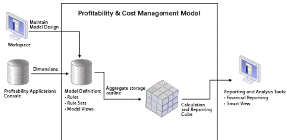
Figure 4-1 Architecture du produit Profitability de grand livre de gestion
