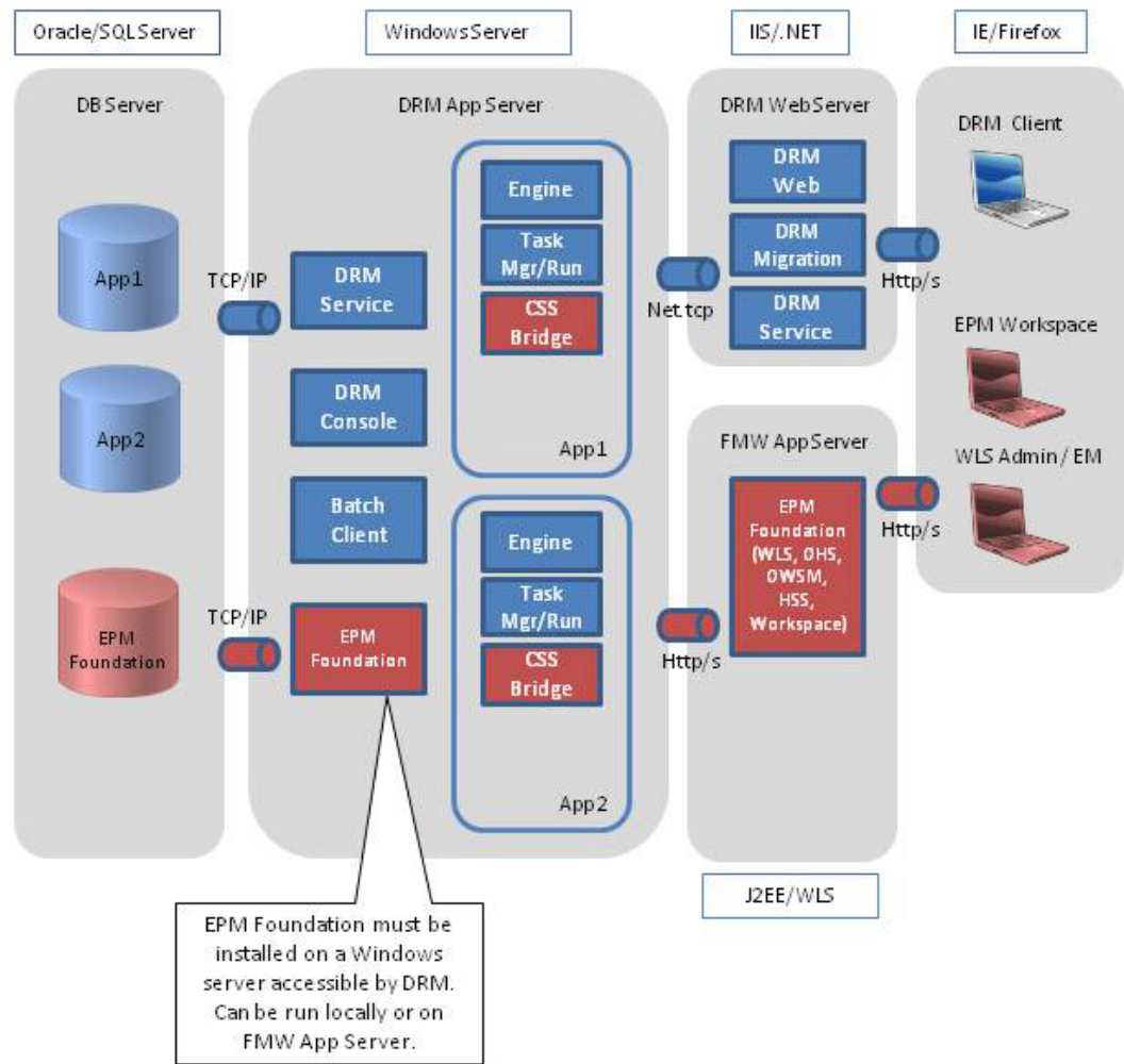
그림 2-2 EPM Foundation을 사용하는 Data Relationship Management
