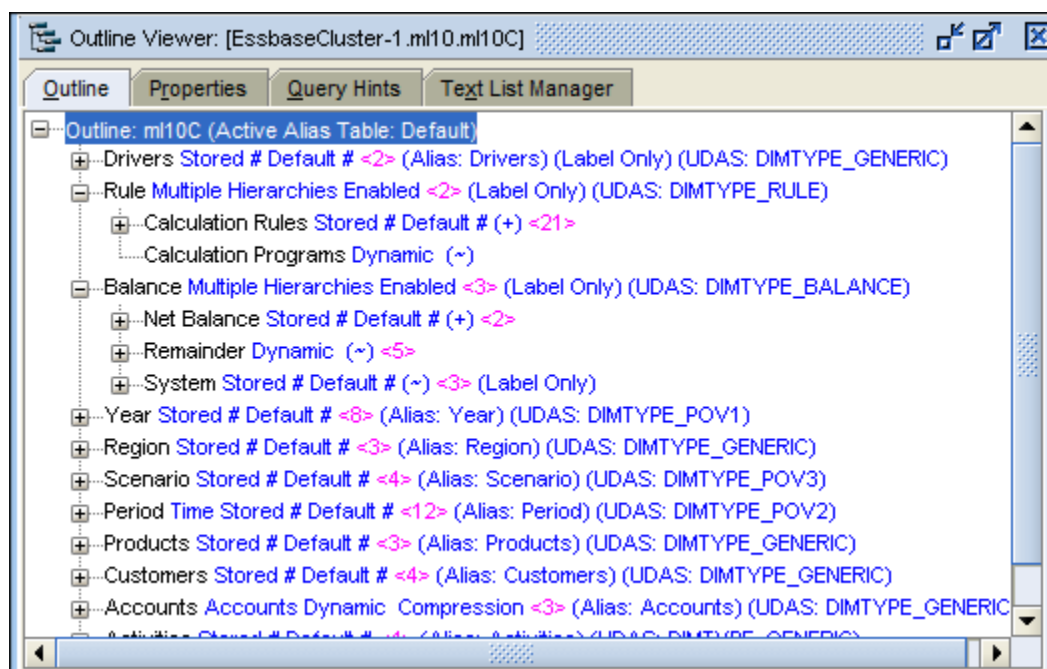
Figura 5-1 Outline do Essbase de um Banco de Dados do Management Ledger
