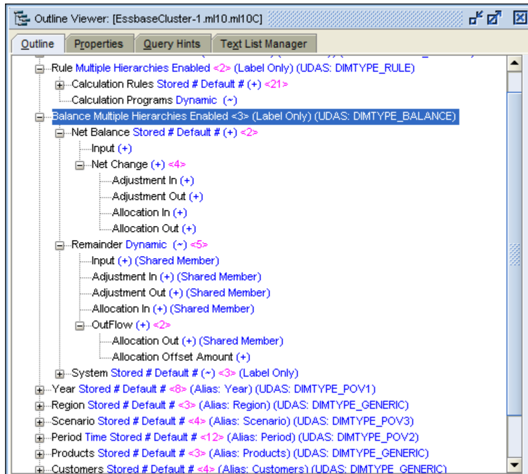
Figura 5-3 Descrição da Dimensão Saldo do Management Ledger
