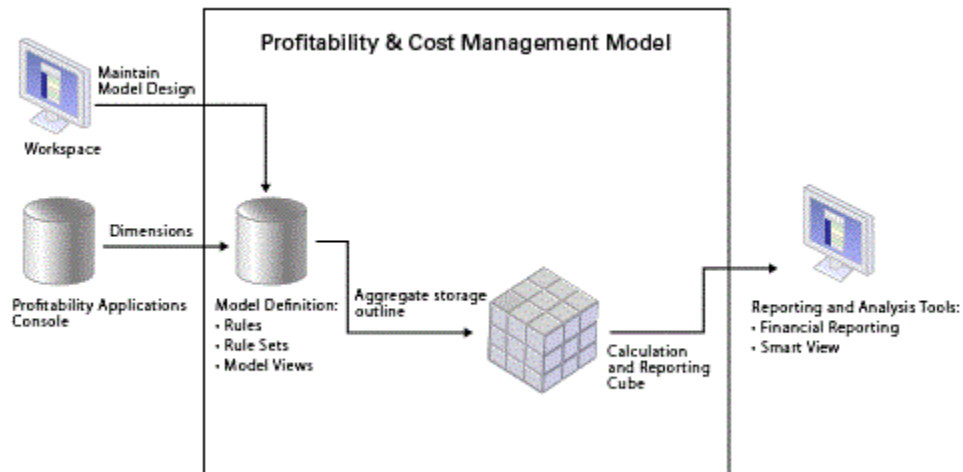
图 4-1 管理分类帐 Profitability 产品体系结构
