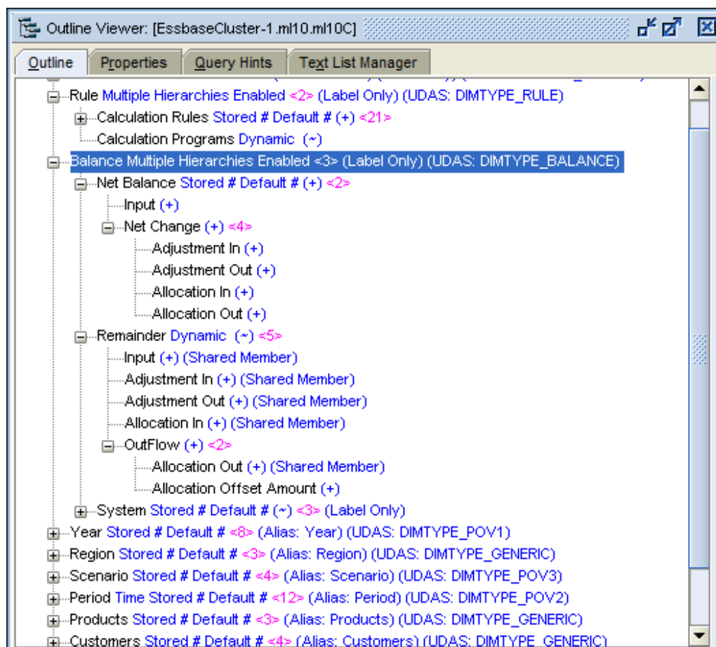
图 5-3 管理分类帐余额维大纲
