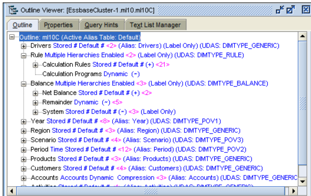
图 5-1 管理分类帐 Profitability 数据库的 Essbase 大纲
