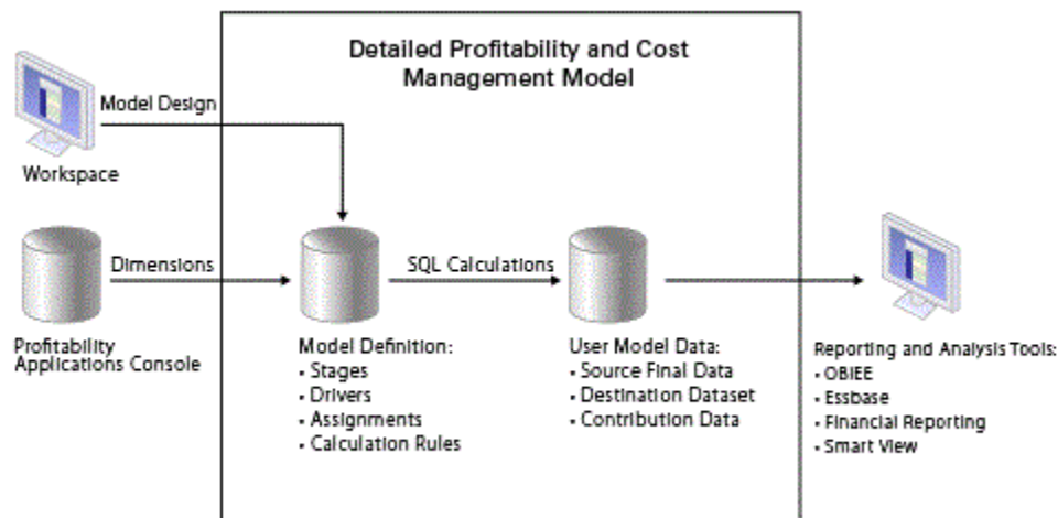
图 7-1 明细 Profitability 体系结构
