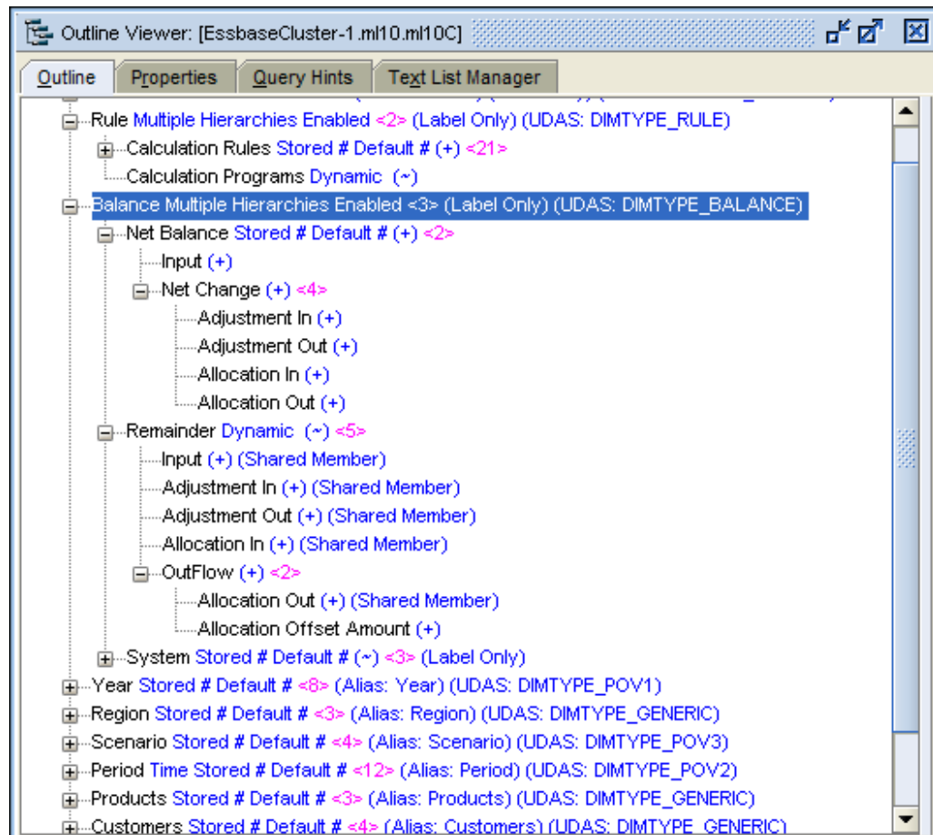
圖 5-3 管理分類帳餘額維度大綱
