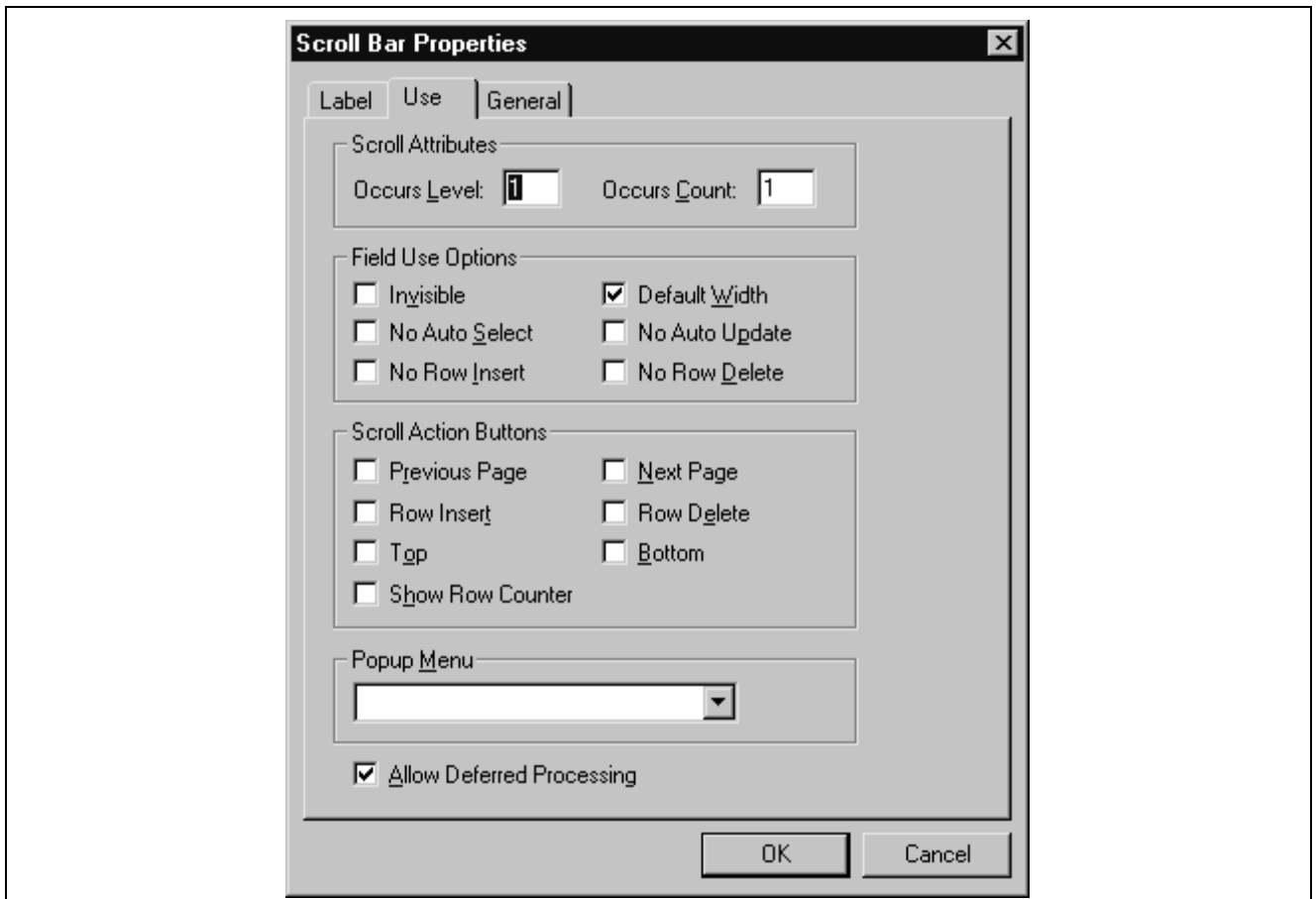
Specifying scroll bar Use
