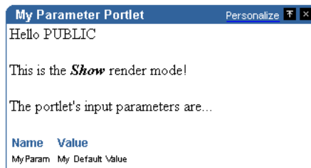
Figure 7-5 Parameter Portlet
