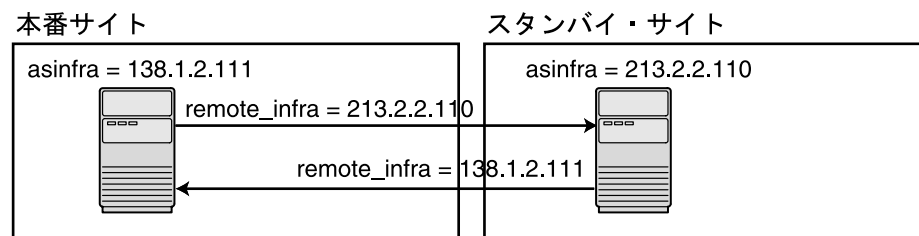
図 6-30 内部 DNS サーバー内の Oracle Data Guard エントリー
