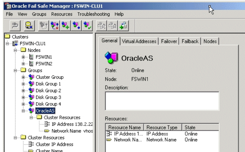
図 6-13 Oracle Fail Safe Manager での新しいグループのリソースの表示
