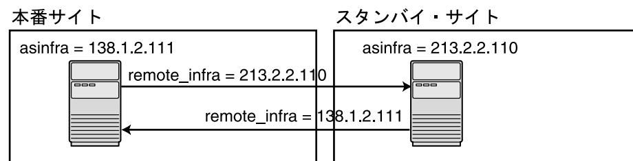
図 6-30 内部 DNS サーバー内の Oracle Data Guard エントリ
