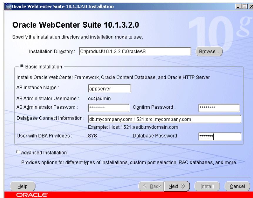
図 4-1 「Oracle WebCenter Suite 10.1.3.2.0 インストレーション」画面
