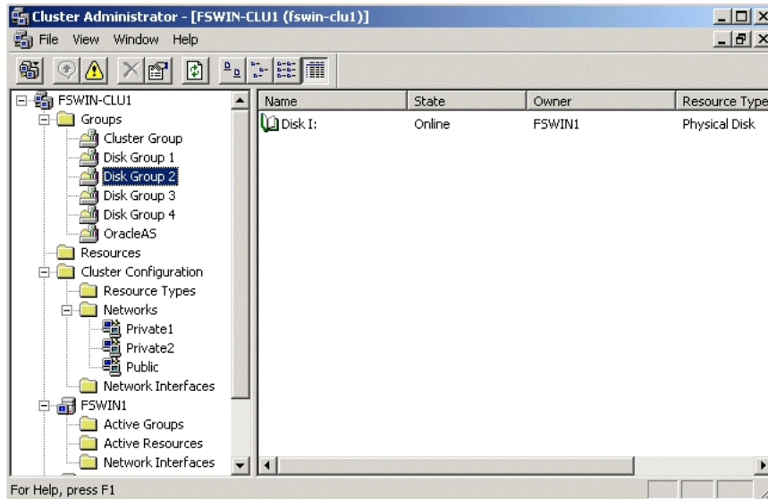
図 6-14 クラスタ・アドミニストレータでの共有ディスクの表示
