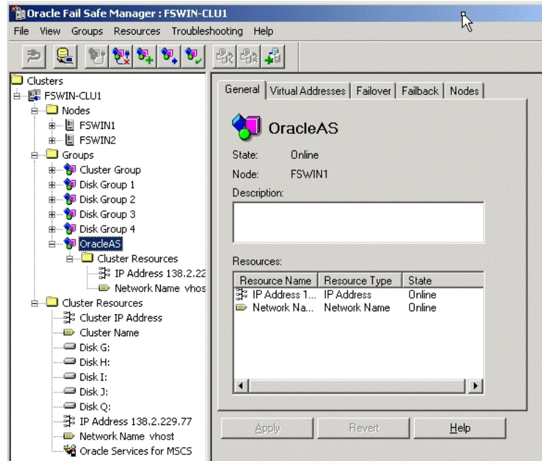
図 6-13 Oracle Fail Safe Manager での新しいグループのリソースの表示
