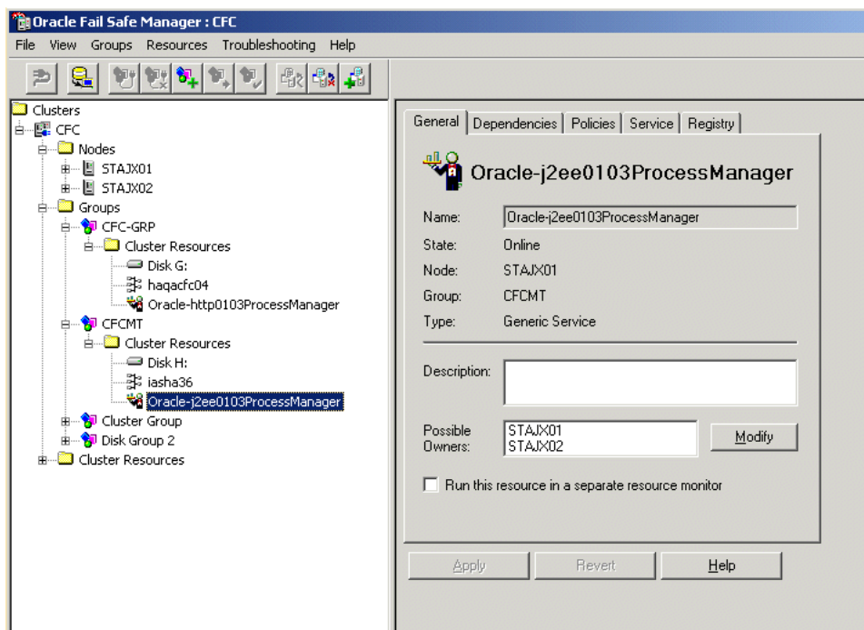
図 6-27 Process Manager サービスをグループに追加した後の Oracle Fail Safe Manager の表示
