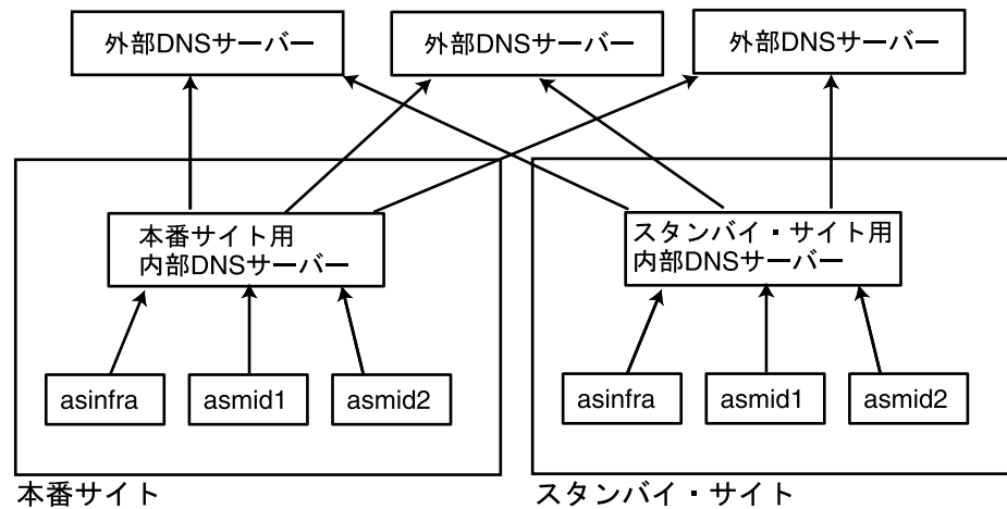
図 6-29 方法 2: DNS サーバーの使用
