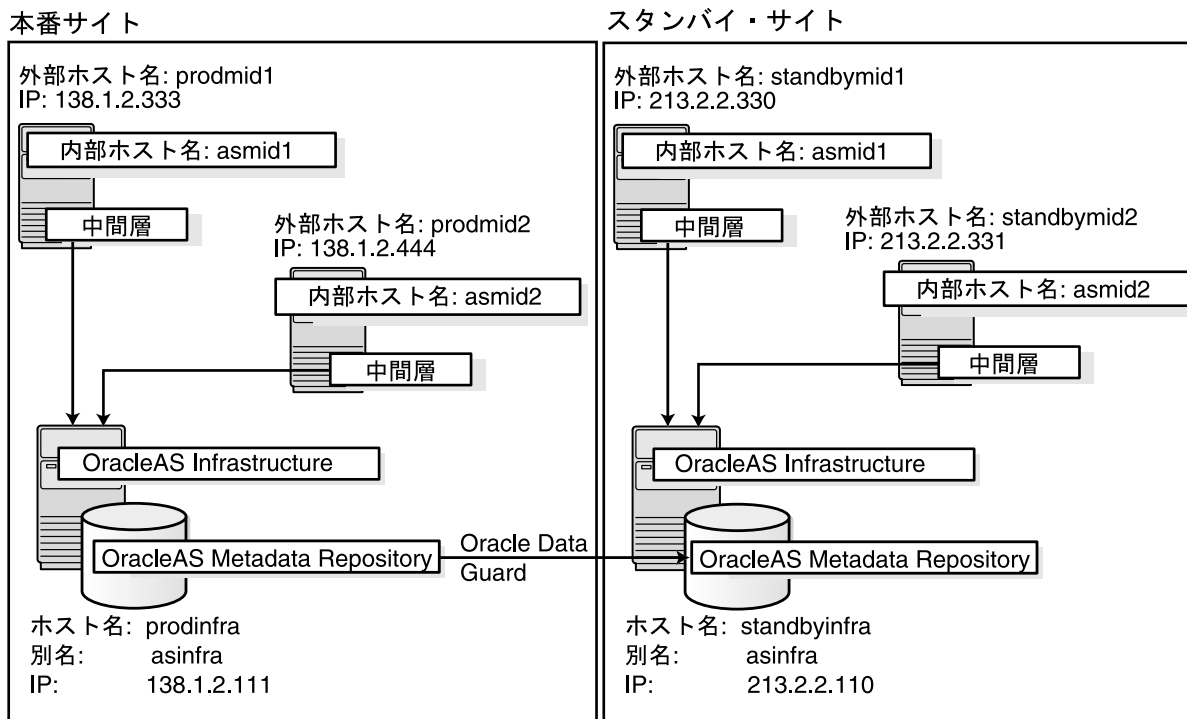
図 6-28 OracleAS Disaster Recovery 環境
