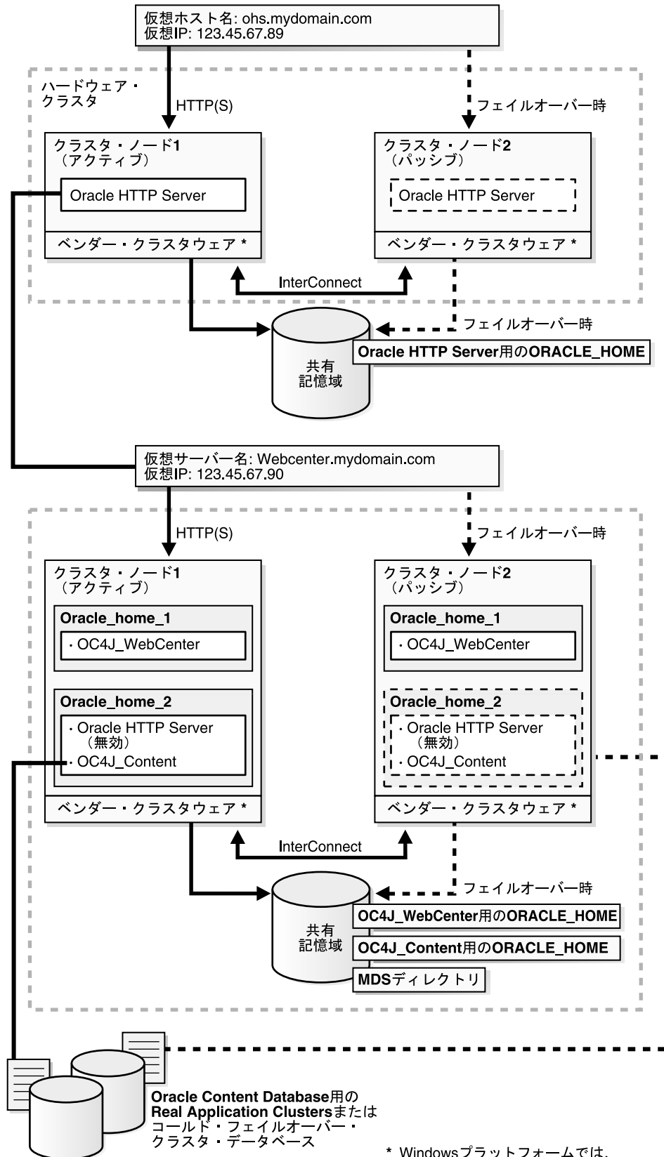
図 6-4 コンポーネントが別々の Oracle ホームにインストールされているアクティブ・パッシブ・トポロジー
