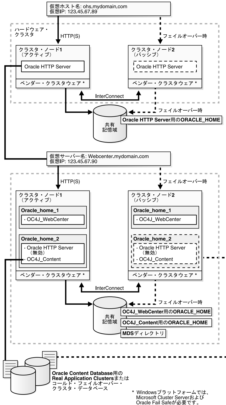
図 6-4 コンポーネントが別々の Oracle ホームにインストールされているアクティブ・パッシブ・トポロジ
