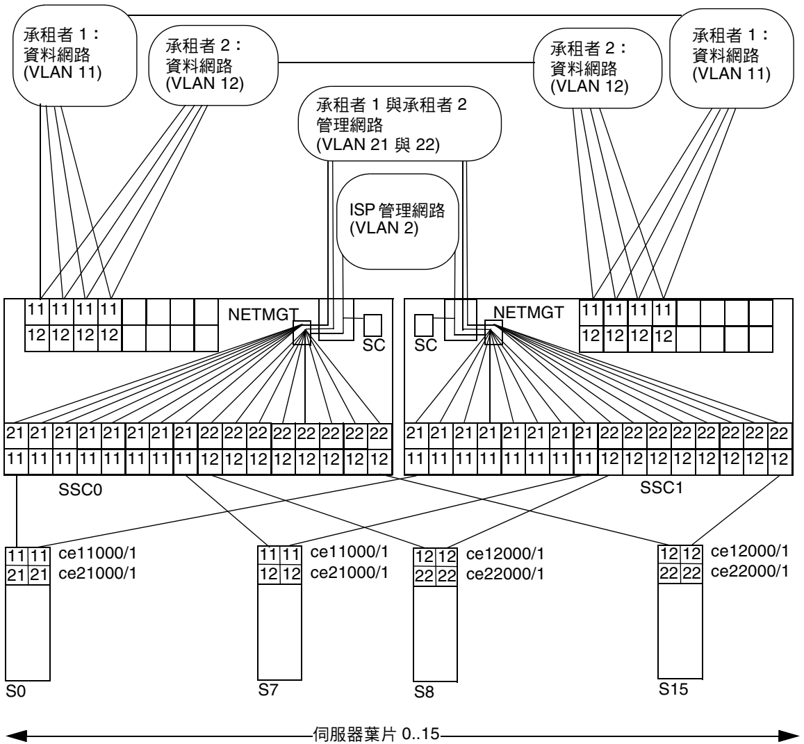
■ 7-2 情境 B：兩個承租者的資料與管理 VLAN 以及共用的對外連接埠
