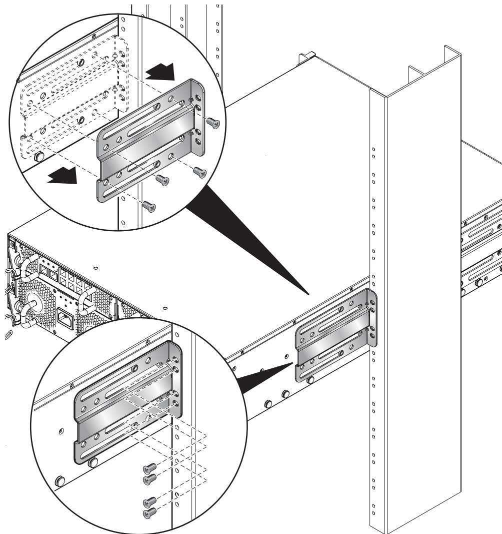
FIGURE 12-17 Retrait des supports arrière
