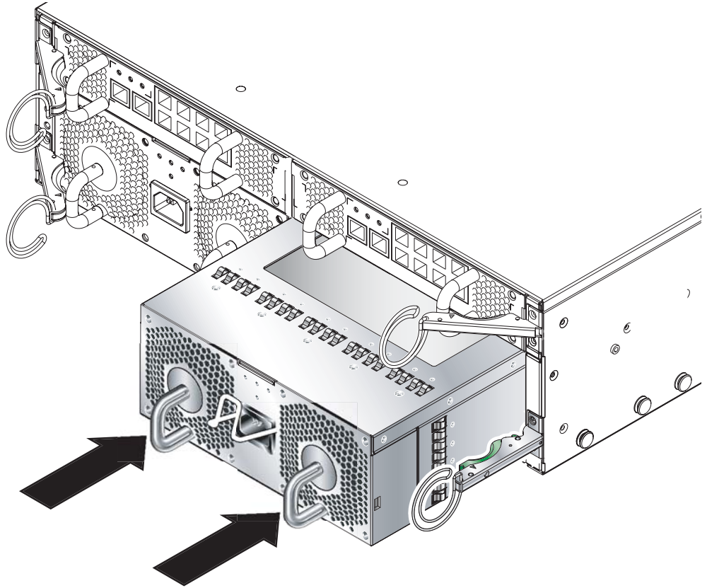
FIGURE 12-14 Engagement du dispositif d'éjection de l'unité d'alimentation
