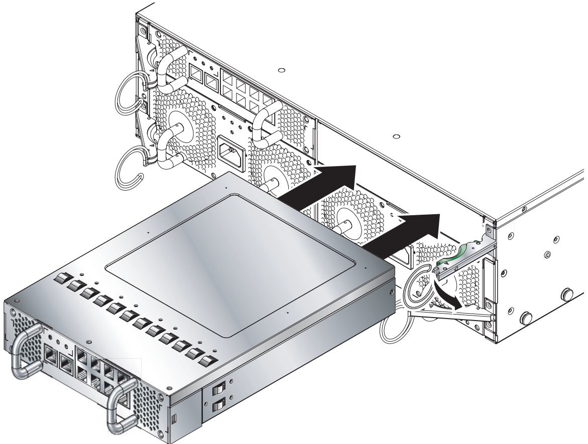
FIGURE 12-9 Alignement de l'unité commutateur/contrôleur système avant son insertion
