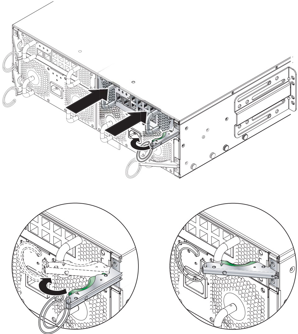
FIGURE 12-11 Fermeture du dispositif d'éjection de l'unité commutateur/contrôleur système
