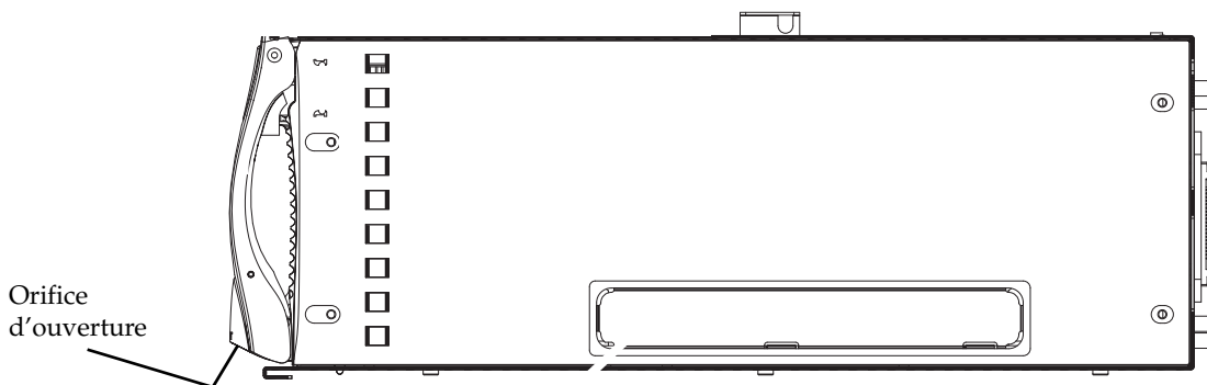
FIGURE 12-4 Mécanisme de verrouillage du serveur Blade
