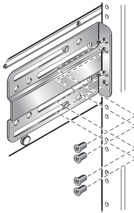
FIGURE 12-18 Retrait des supports avant de l'armoire
