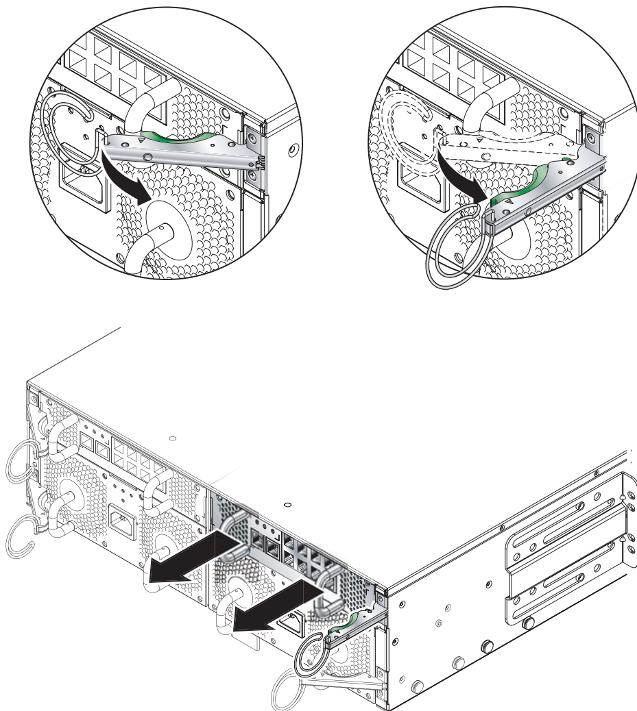
FIGURE 4-12 Levier d'éjection du SSC
