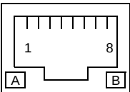
FIGURE 5-6 Port de gestion de réseau 10 / 100BASE-T
