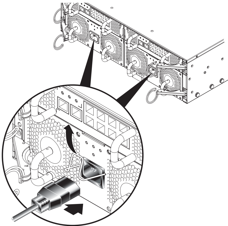
FIGURE 5-2 Insertion des cordons d'alimentation IEC
