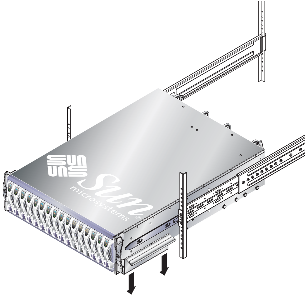
FIGURE 3-7 Retrait de la poignée de levage amovible (armoie 19" à quatre colonnes)
