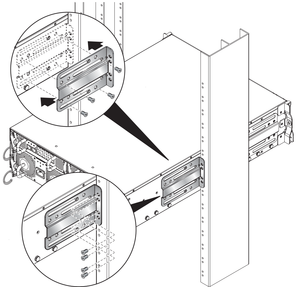
FIGURE 3-12 Fixation des équerres arrière (armoire 19" à deux colonnes)
