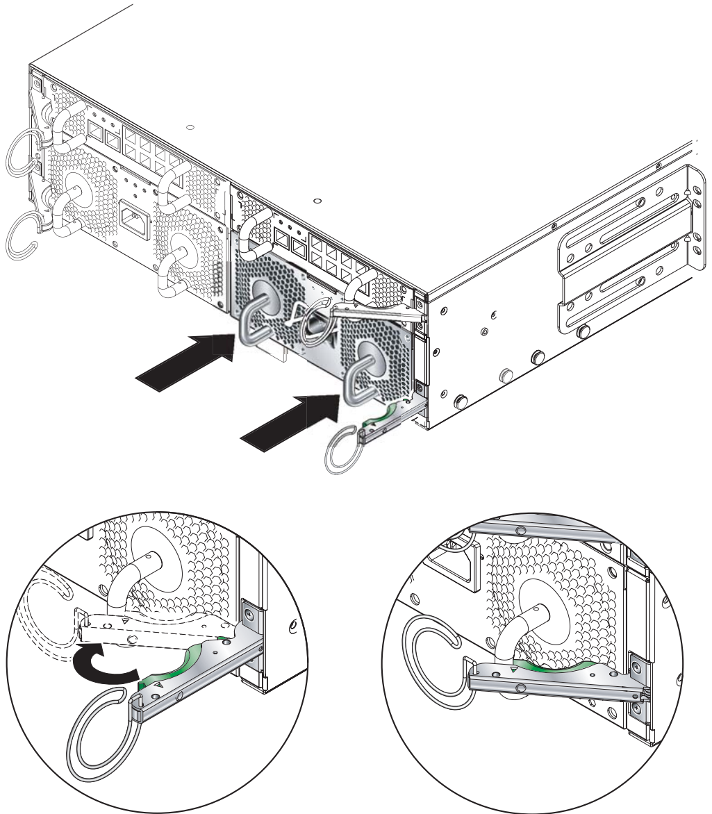
FIGURE 4-11 Fermeture du levier d'éjection du PSU
