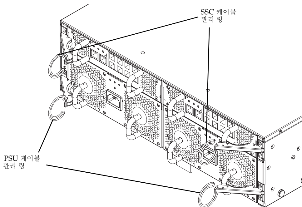
그림 5-8 후면의 케이블 관리 링
