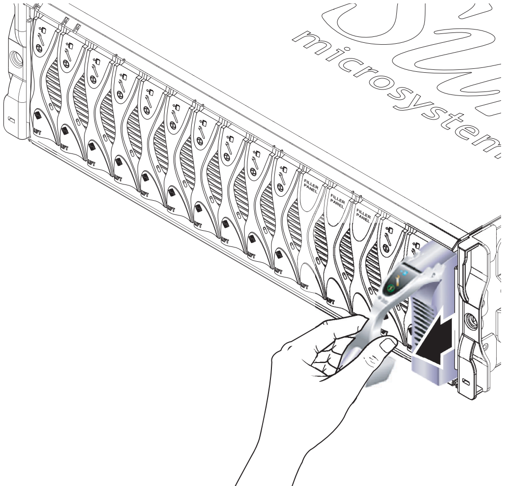
그림 4-2 블레이드 꺼내기
