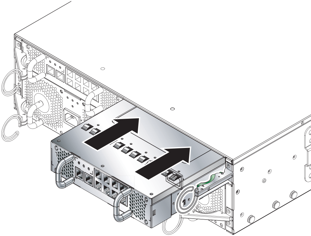
그림 4-15 SSC 삽입
