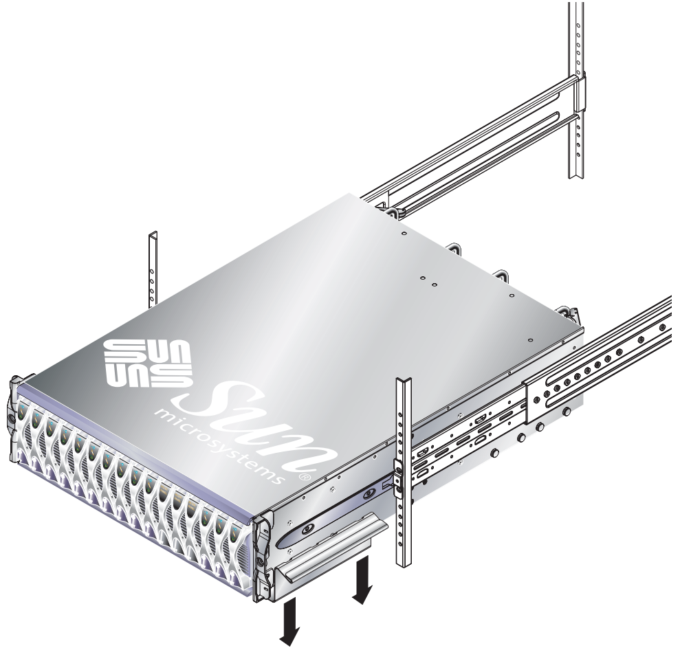
그림 3-7 운반 손잡이 제거(19인치, 4기둥 랙)
