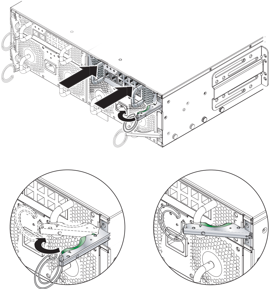
그림 4-16 SSC 방출 레버 닫기
