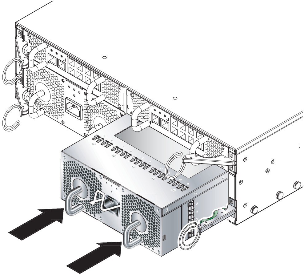
그림 4-10 시스템 채시 속으로 PSU 밀어넣기
