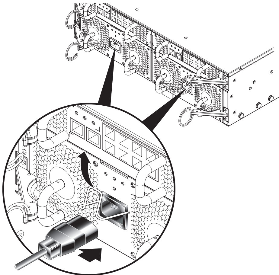
그림 5-2 IEC 전원 코드 삽입
