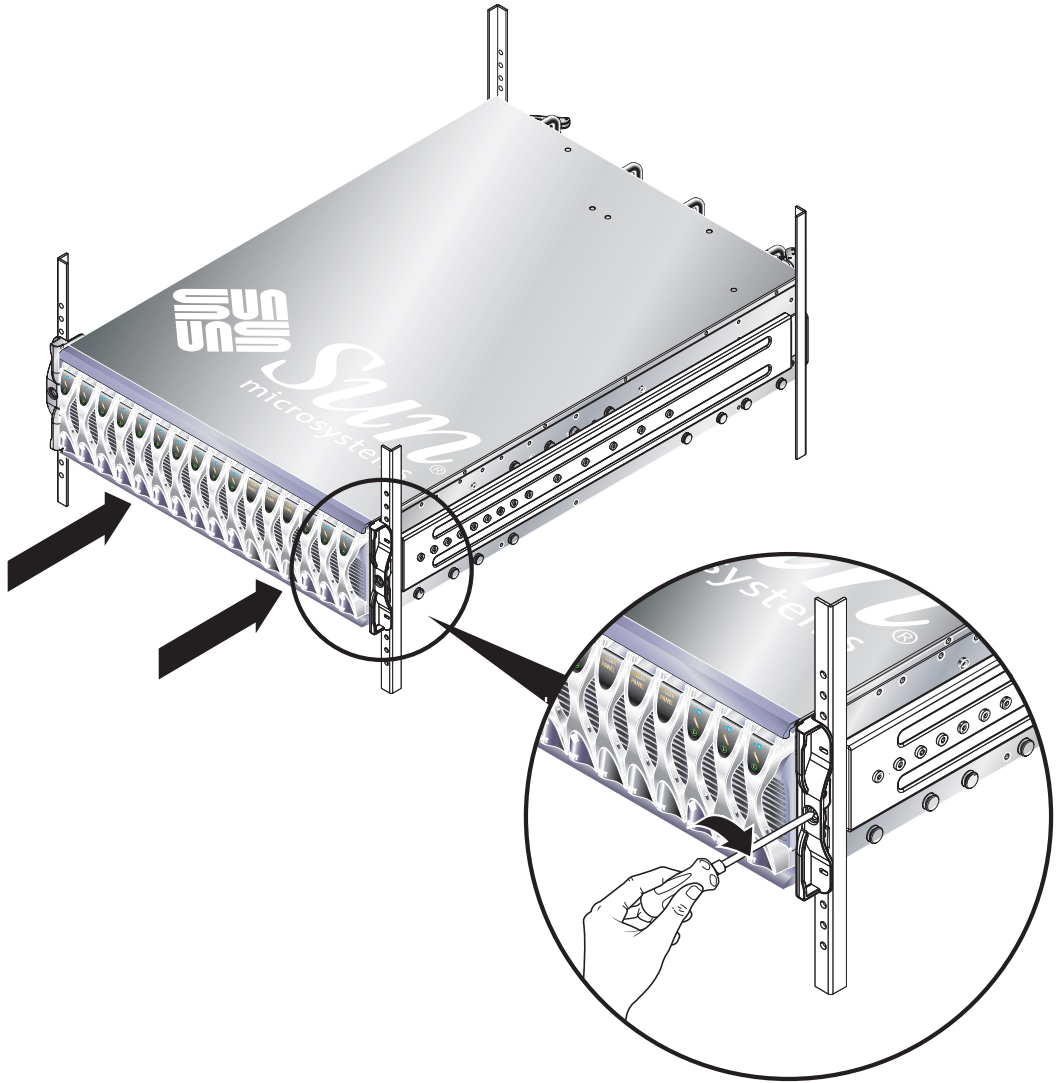
그림 3-8 고정 나사 조이기(19인치, 4기둥 랙)
