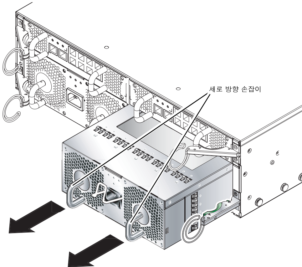
그림 4-8 시스템 채스에서 PSU 꺼내기
