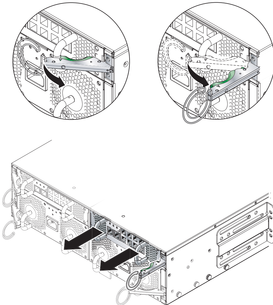
그림 4-12 SSC 방출 레버
