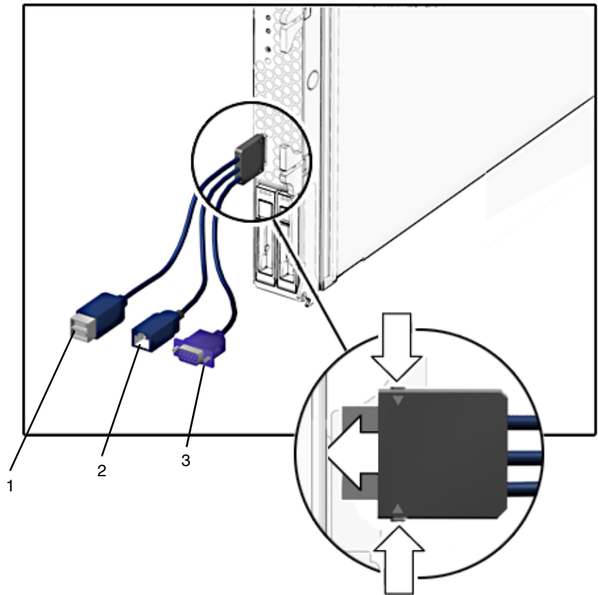
圖 2 硬體鎖纜線
