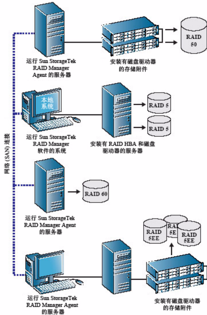
图 1-4 多系统存储空间配置
