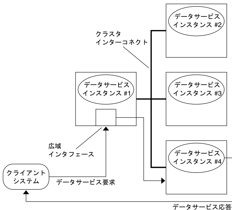
図 3-8 スケーラブルサービスの構造
