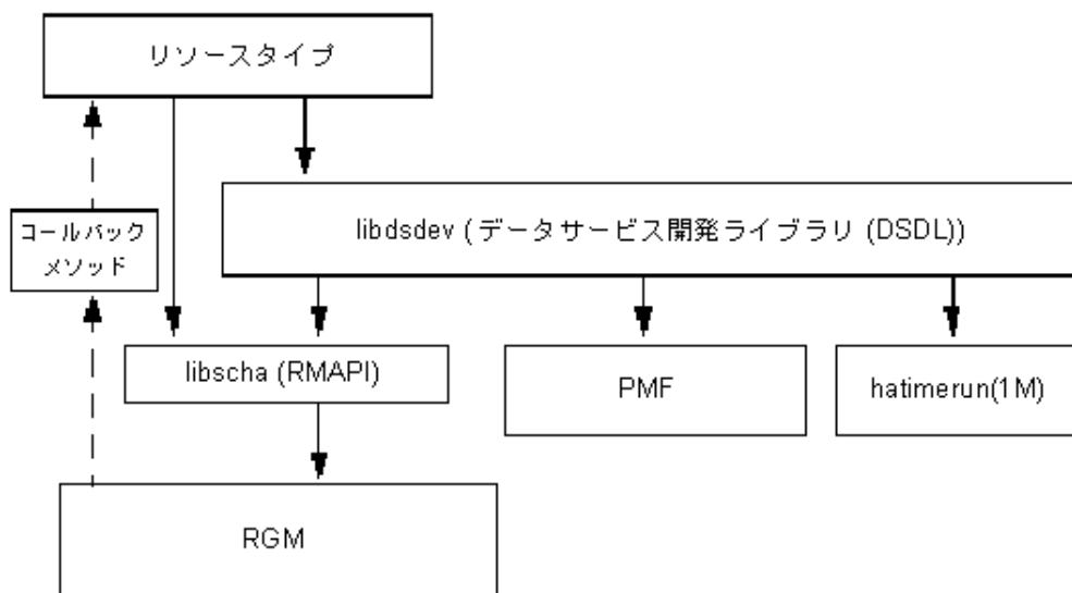
図 1-1 プログラミングアーキテクチャ
