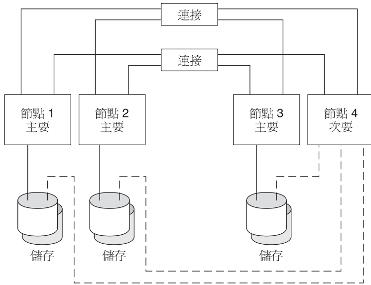
圖 2-5 N+1 拓模架構
