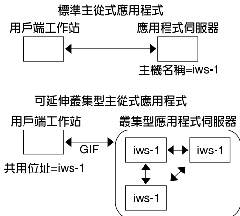
圖 3-6 固定主機名稱與共用位址
