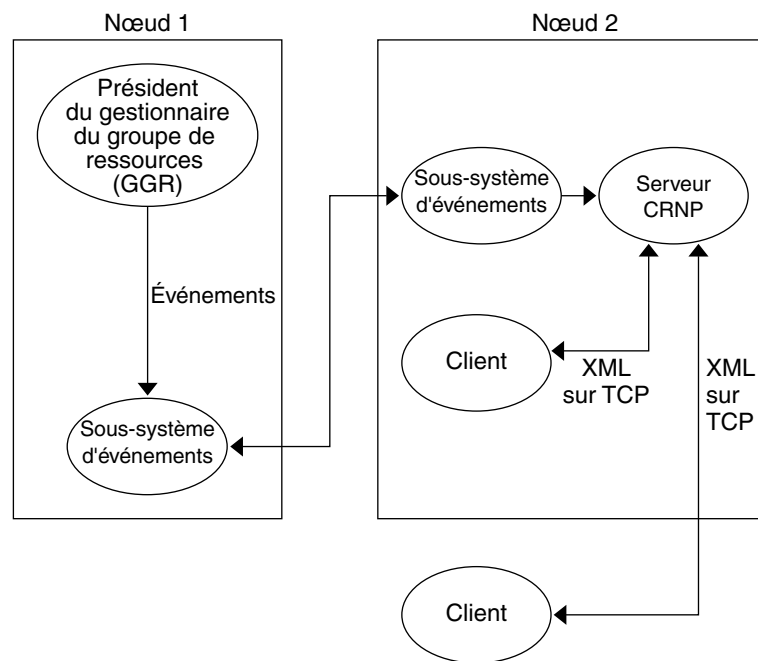
FIGURE 12-1 Fonctionnement du protocole CRNP
