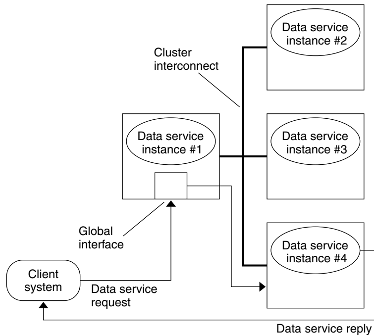
图 3-3 可伸缩数据服务体系结构
