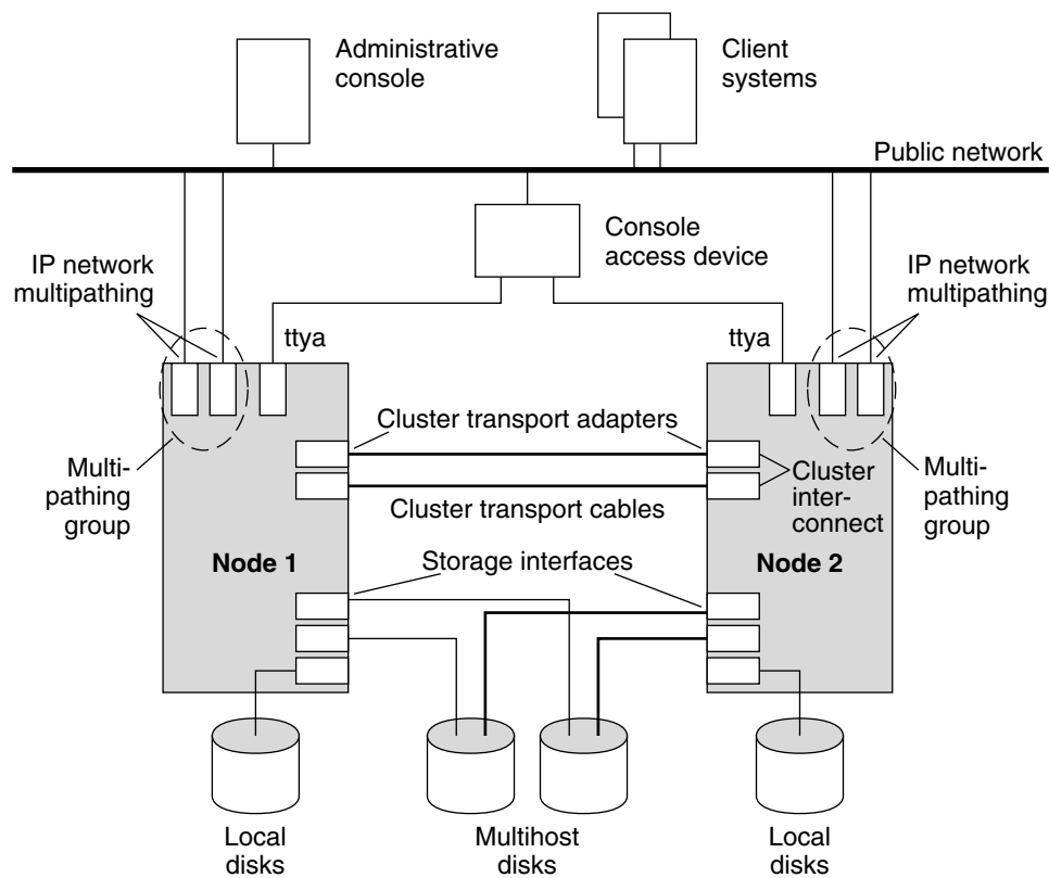
图 3-1 Sun Cluster 硬件组件
