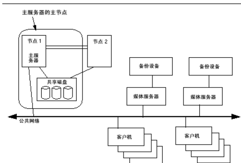
图 1 Sun Cluster HA for NetBackup 支持的配置
