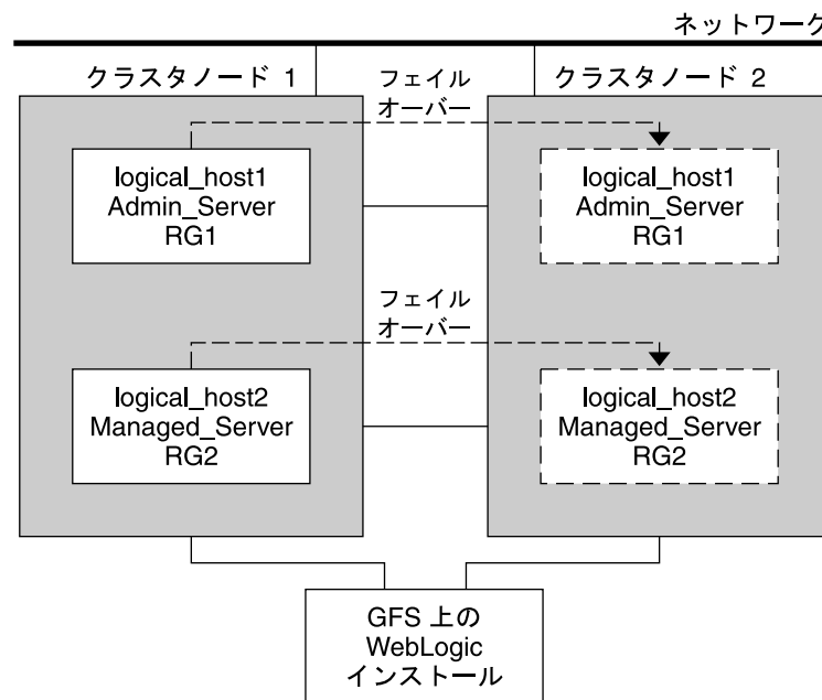
図 1 Sun Cluster HA for BEA WebLogic Server によるシンプルな構成
