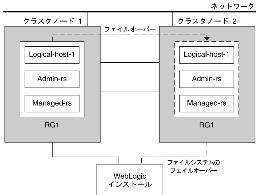
図 2 Sun Cluster HA for BEA WebLogic Server ファイルシステムのフェイルオーバー構成
