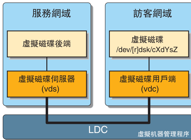
圖 5-1 搭配 Logical Domains 的虛擬磁碟
