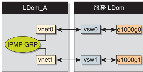
圖 6-1 連線至個別虛擬交換器實例的兩個虛擬網路
