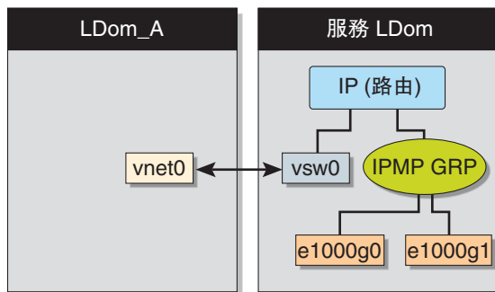
圖 6-3 配置為 IPMP 群組之一部分的兩個網路介面
