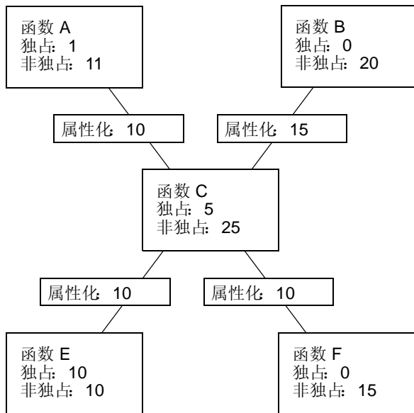
图 2-1 描述独占、非独占和属性衡量标准的调用树
