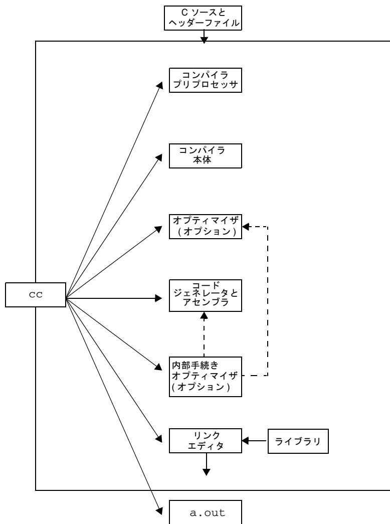
図 1-1 C コンパイルシステムの構成
