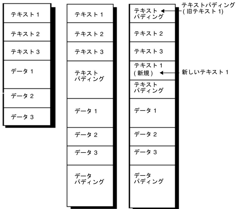
図 4-1 インクリメンタルリンク処理の例
