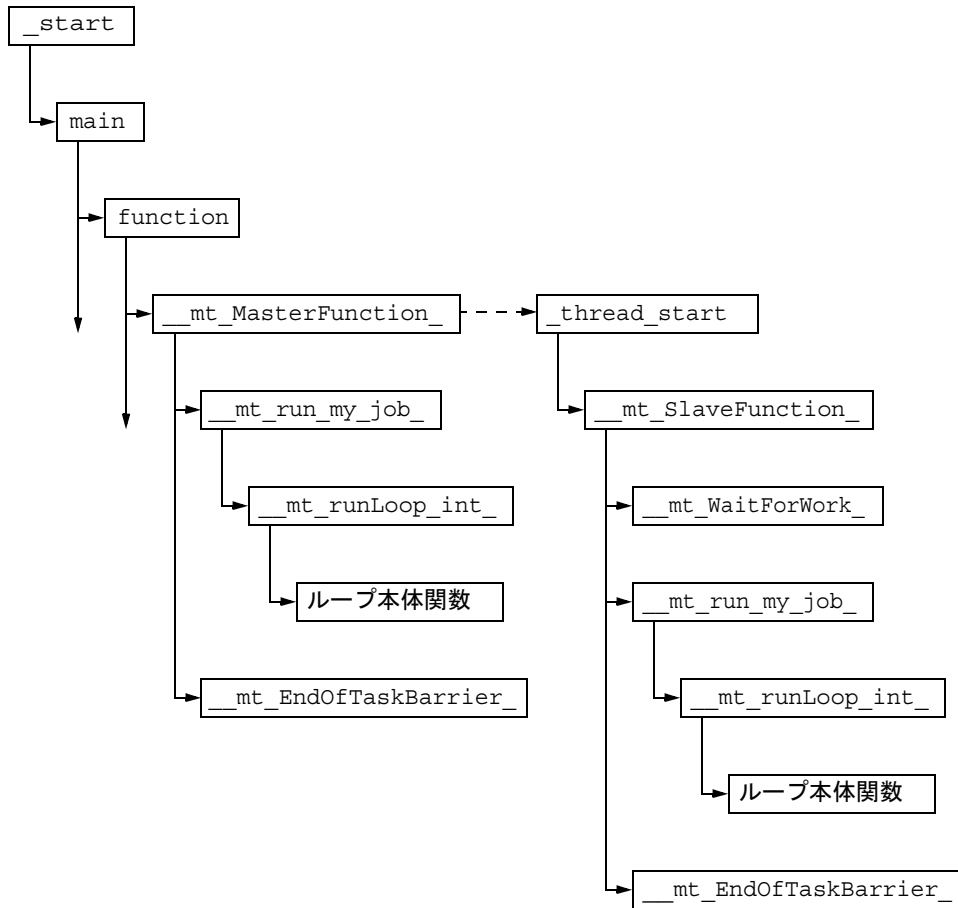
図 5-1 Parallel Do または Parallel For 構造を含むマルチスレッドプログラムの呼び出しツリー
