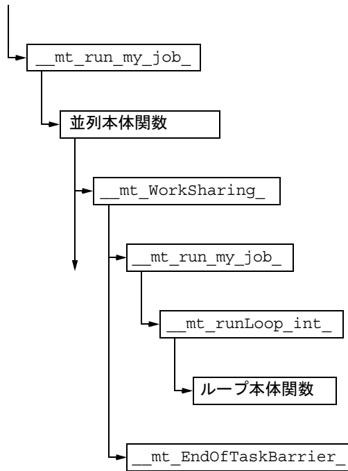
図 5-2 Worksharing Do または Worksharing For 構造を含む並列領域の呼び出しシーケンス
