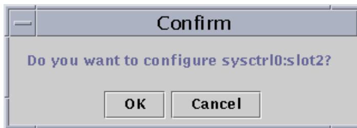
그림 5 확인 대화상자
