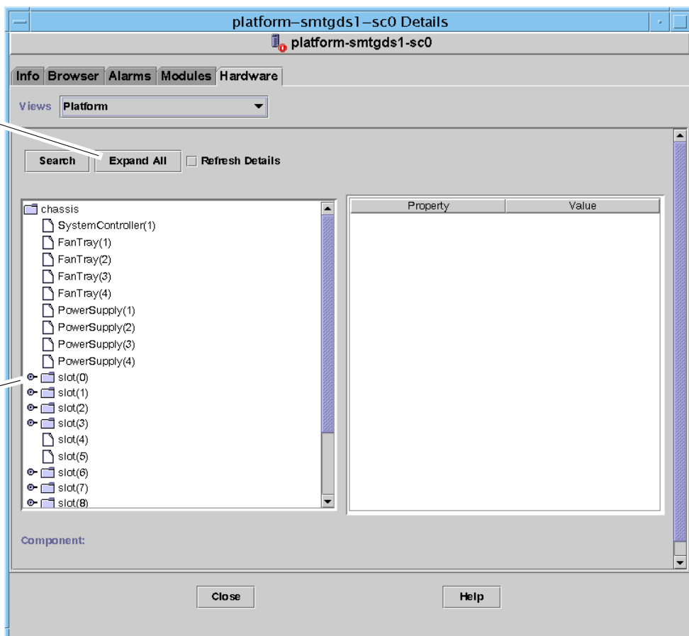
圖 3-21 邏輯視區
