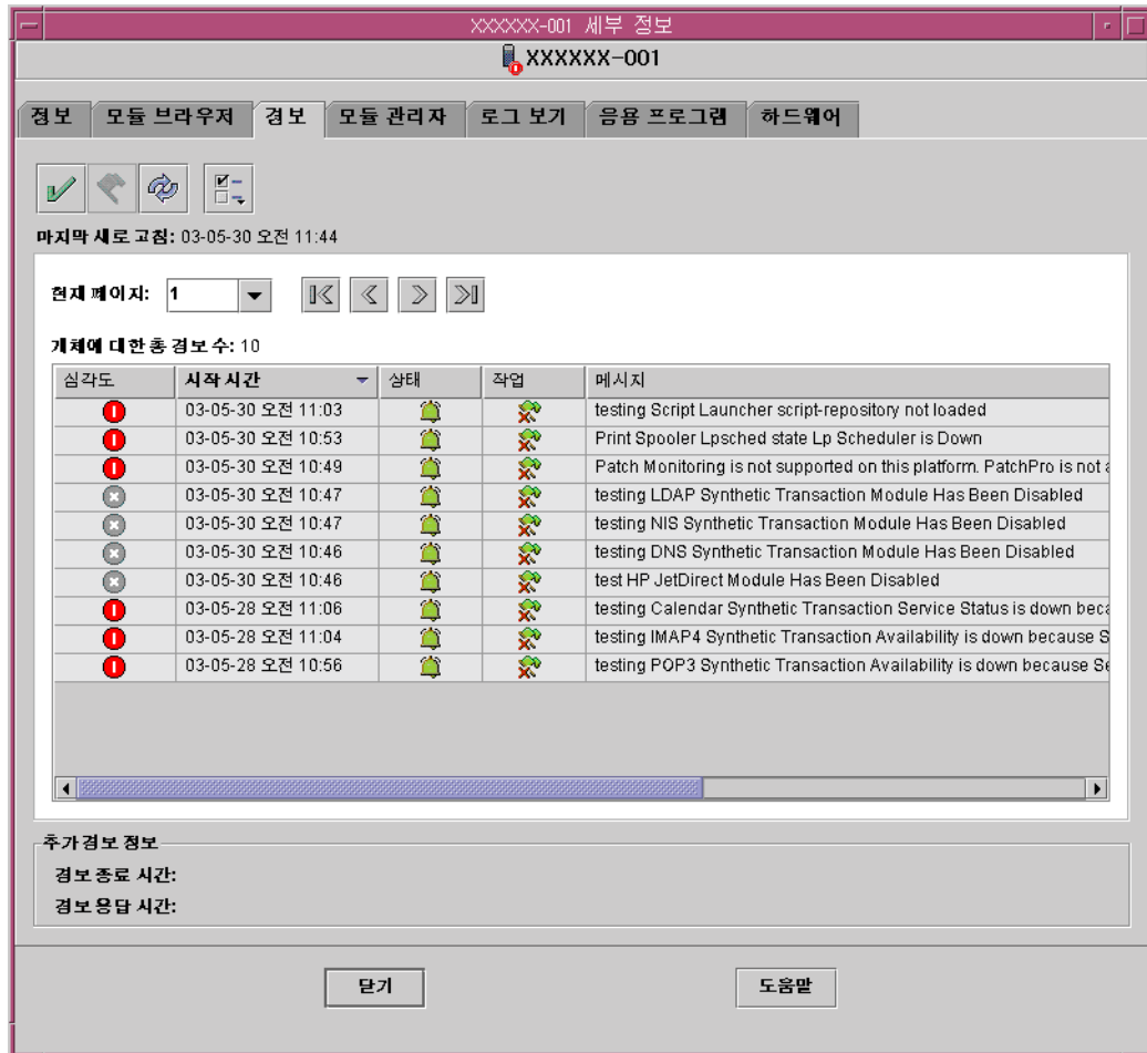
그림 12-2 정보 세부 정보 창
