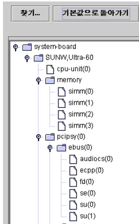
그림 6-7 논리적 뷰의 확장된 구성 요소 토폴로지
