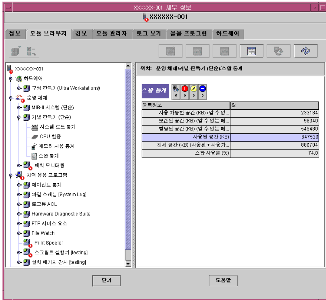
그림 12-1 세부 정보 창의 스왑 통계 정보
