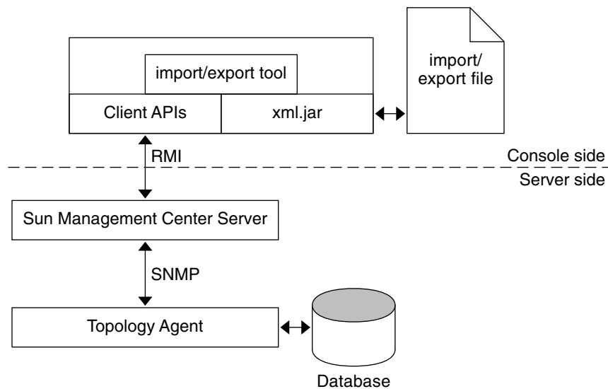
그림 19-1 토폴로지를 가져오고 내보내는 소프트웨어 구조
