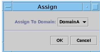
그림 3-5 Assign(지정) 패널
