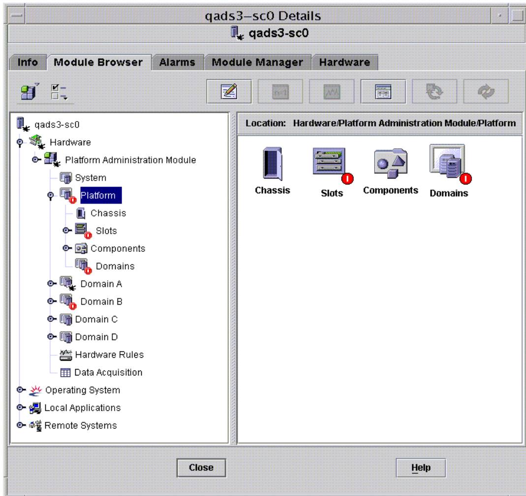
그림 3-4 플랫폼 테이블
