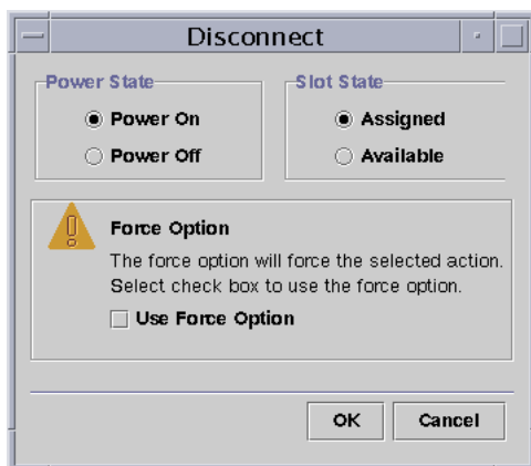
그림 5-3 Disconnect(단절) 패널
