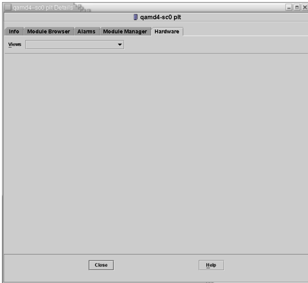
그림 3-19 Hardware(하드웨어) 탭
