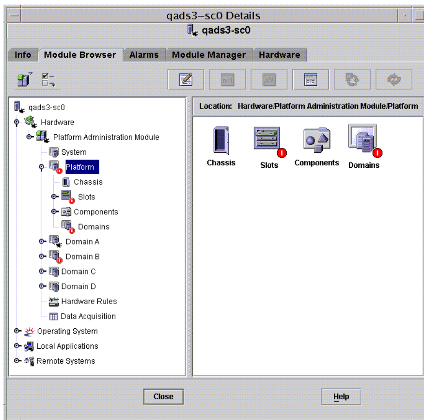
圖 3-1 Sun Fire 中階系統平台物件詳細資訊視窗
