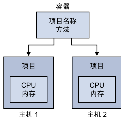
图 3-1 容器和项目
