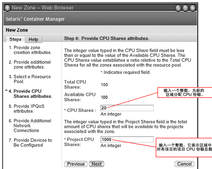
图 3-10 区域份额
