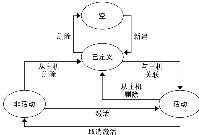
图 3-2 项目状态
