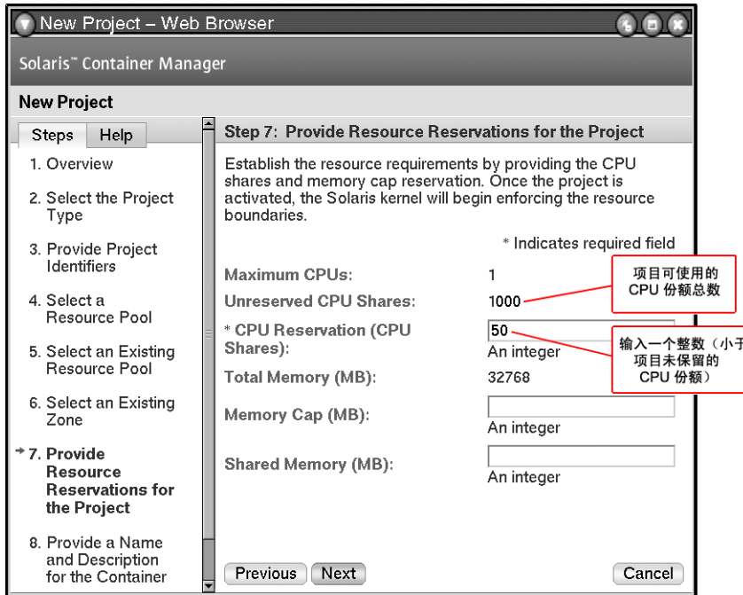
图 3-9 CPU 份额
