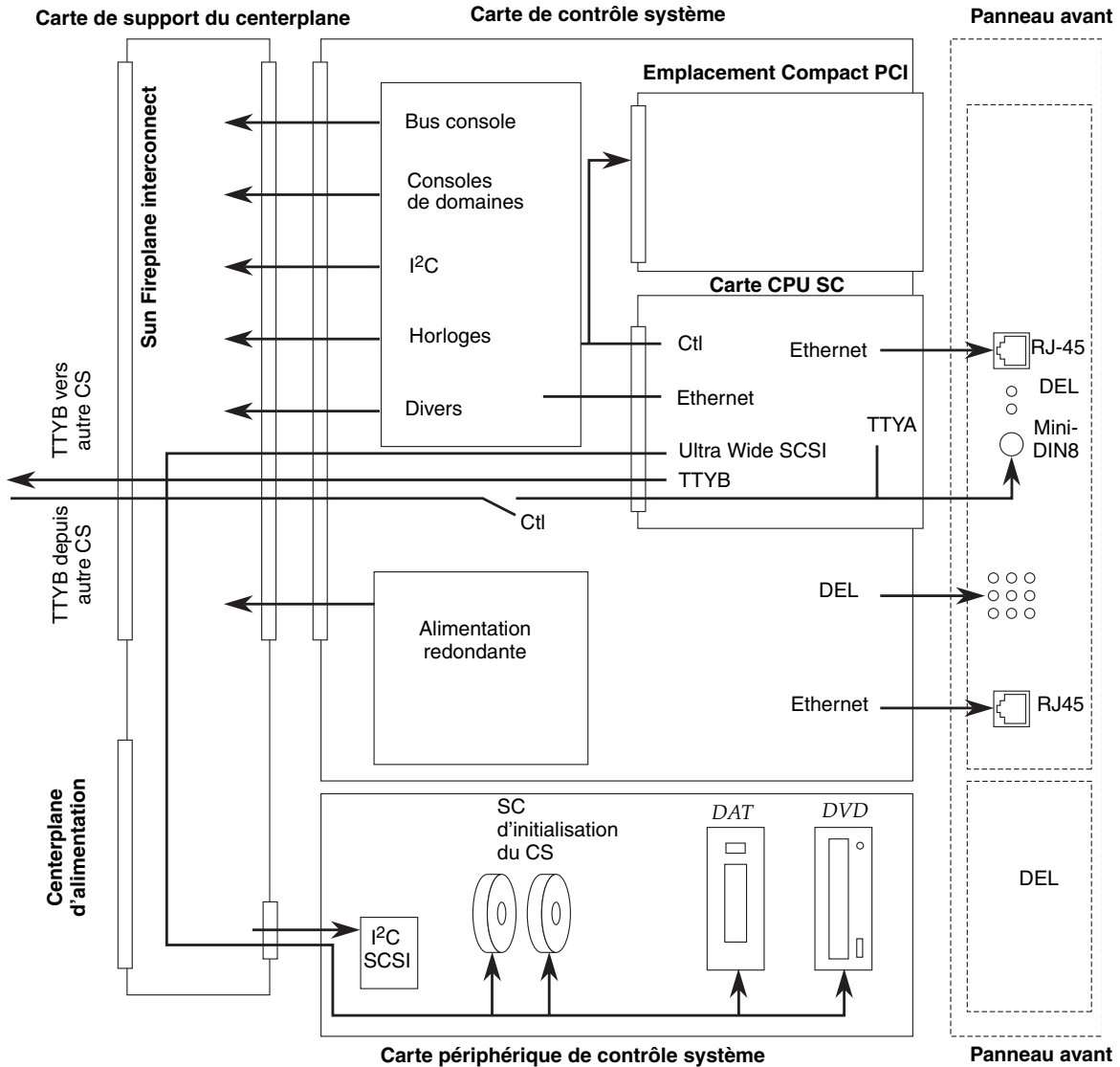
FIGURE 5-6 Configuration de cartes contrôleur système
