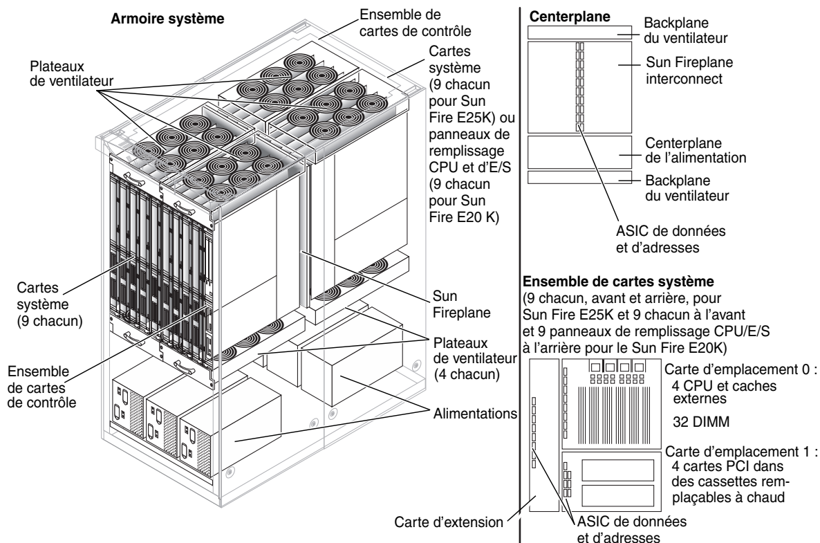
FIGURE 5-1 Principaux composants des Systèmes Sun Fire E25K/E20K
