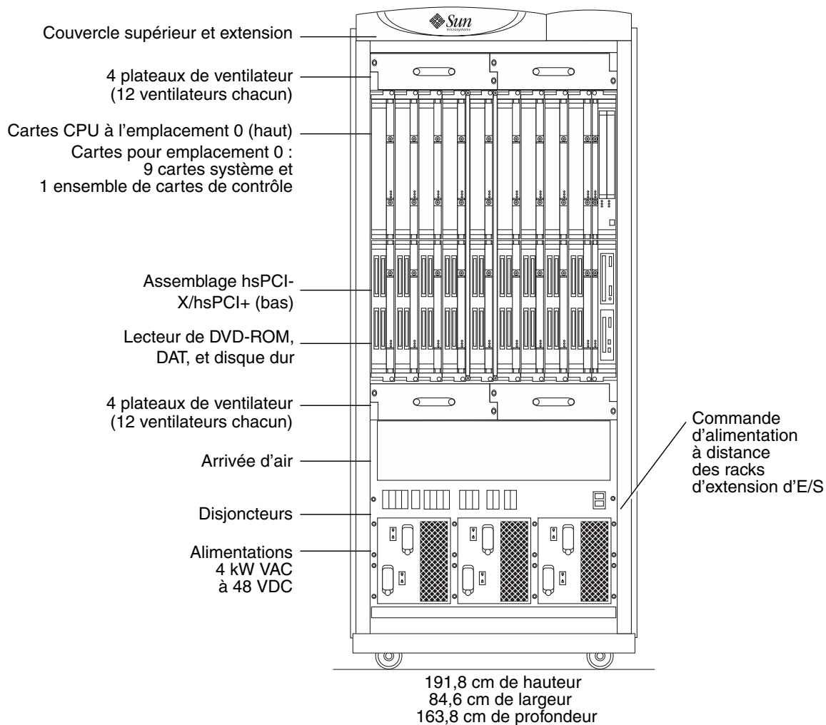
FIGURE 5-2 Armoires des Systèmes Sun Fire E25K/E20K - vue de face
