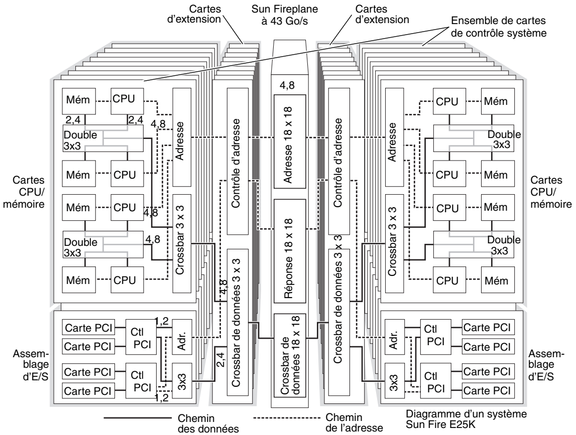
FIGURE 4-1 Interconnexion d'un système Sun Fire E25K/E20K
