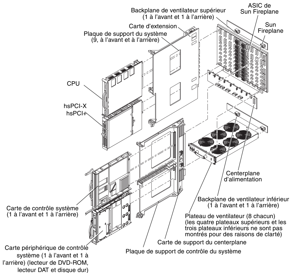
FIGURE 5-3 Sun Fireplane Interconnect et autres composants
