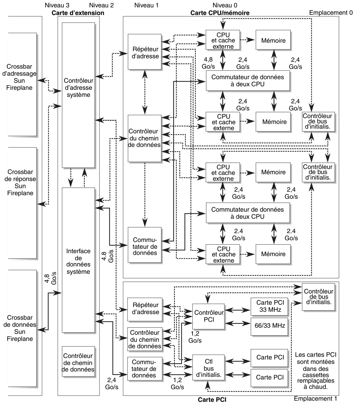
FIGURE 5-4 Diagramme représentant les ensembles de cartes
