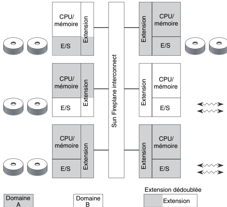
Diagramme illustrant le système Sun Fire 25K
