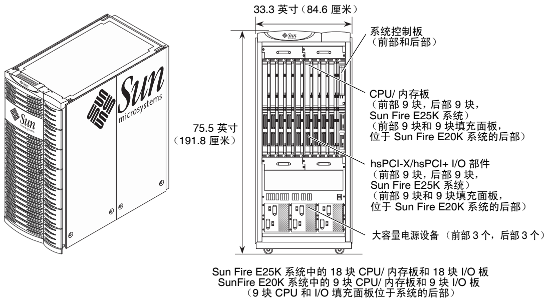
图 1-1 Sun Fire E25K/E20K 系统
