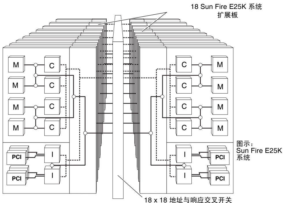
图 1-2 Sun Fireplane 互连体系结构
