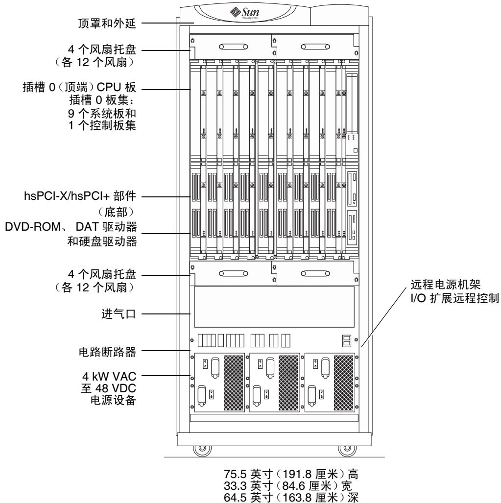
图 5-2 Sun Fire E25K/E20K 系统机箱 - 前视图
