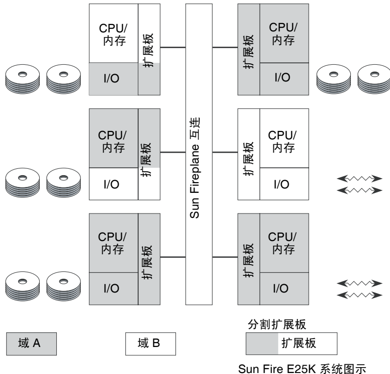
图 2-1 具有一些分割板集的域配置实例
