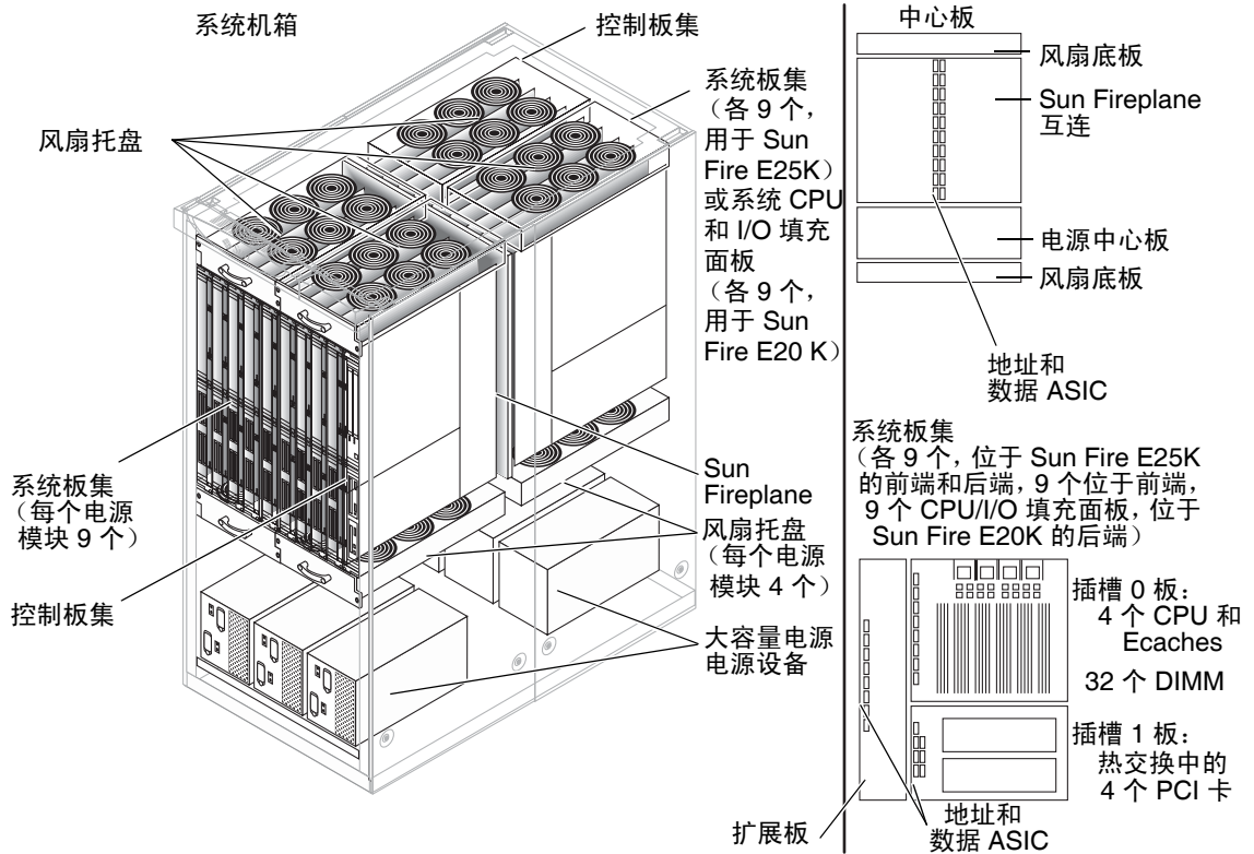
图 5-1 Sun Fire E25K/E20K 系统主要部件
