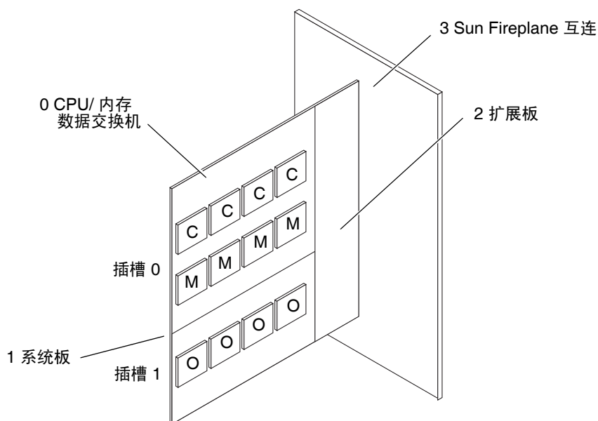
图 4-2 Sun Fire E25K/E20K 系统数据传输互连级别
