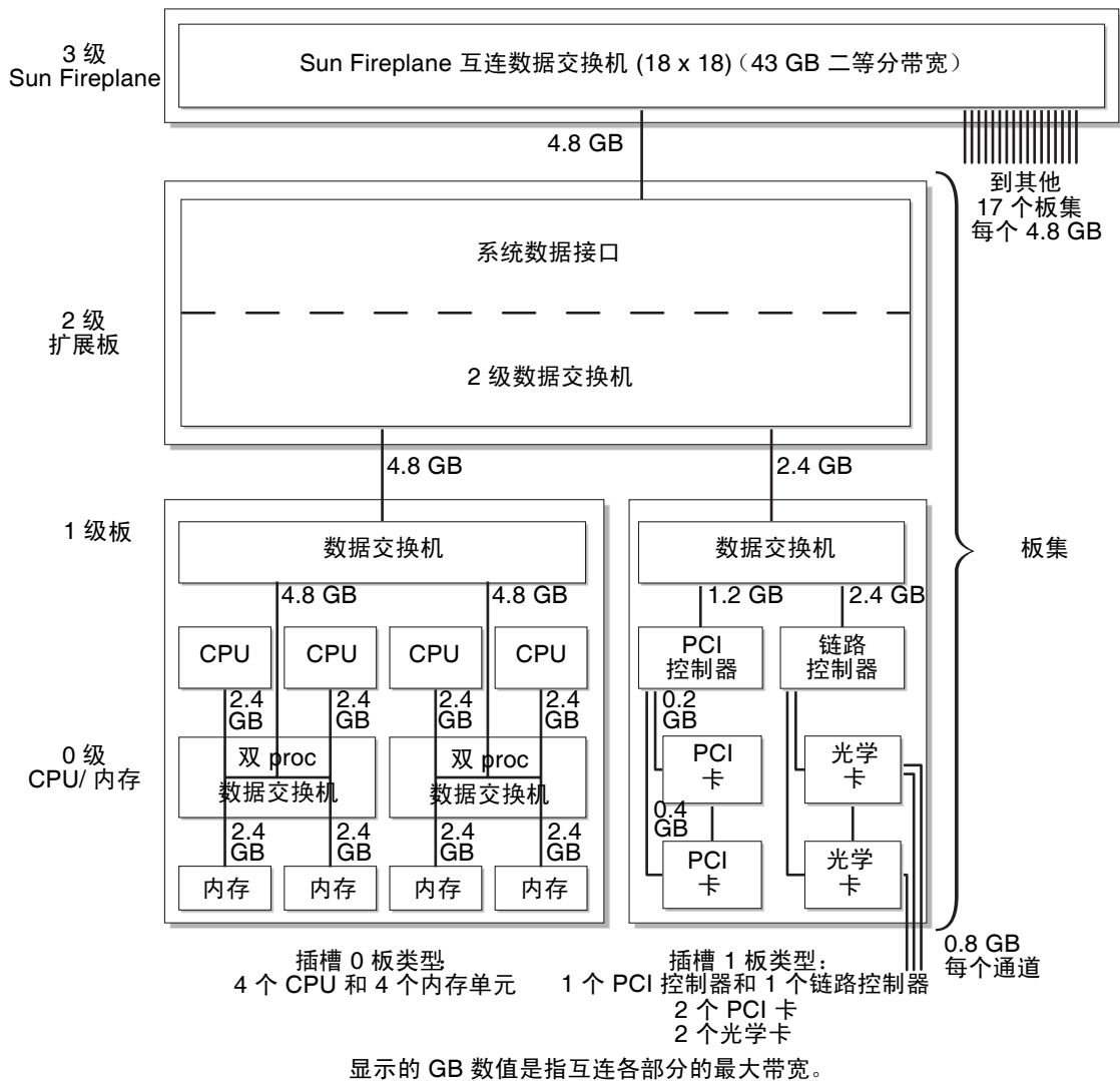
图 4-4 数据互连级别
