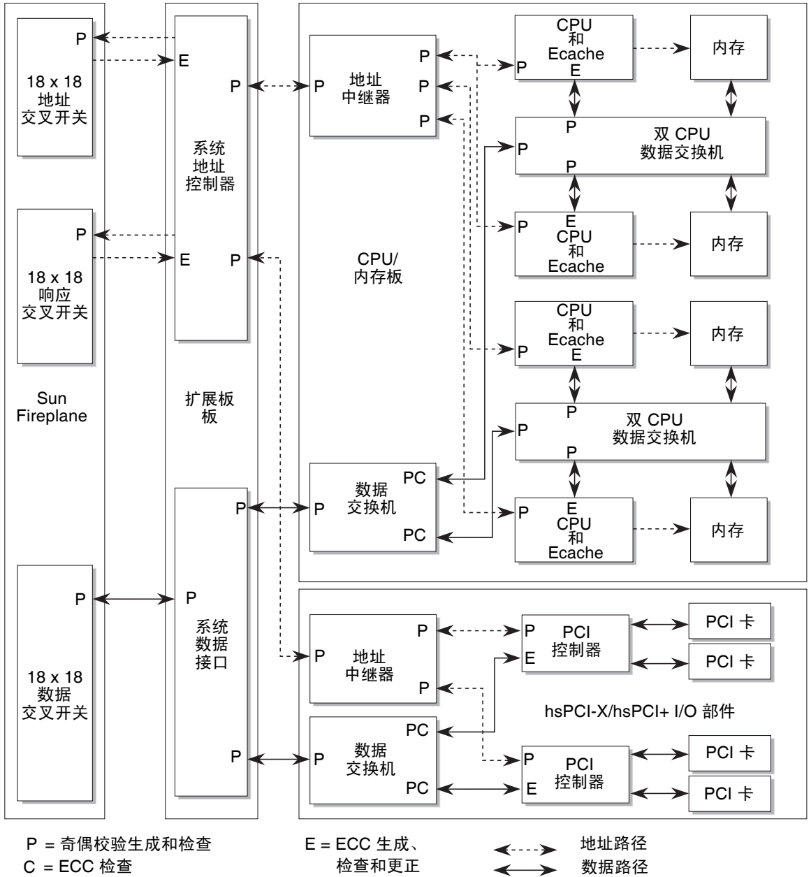
图 3-2 互连 ECC 和奇偶校验检查
