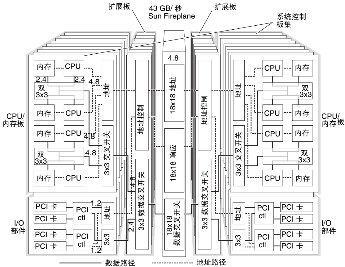
Sun Fire E25K 系统图示
