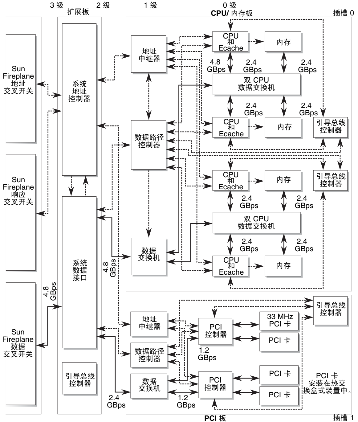
图 5-4 板集框图
