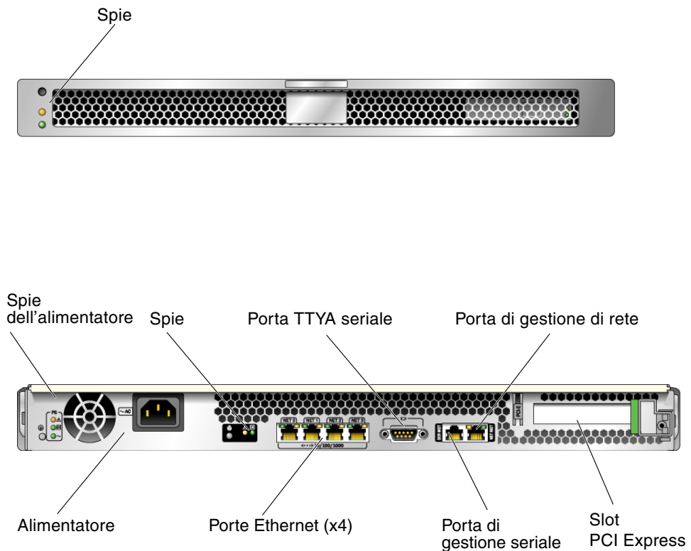
FIGURA 3 Pannello anteriore e posteriore del server Sun SPARC Enterprise T1000
