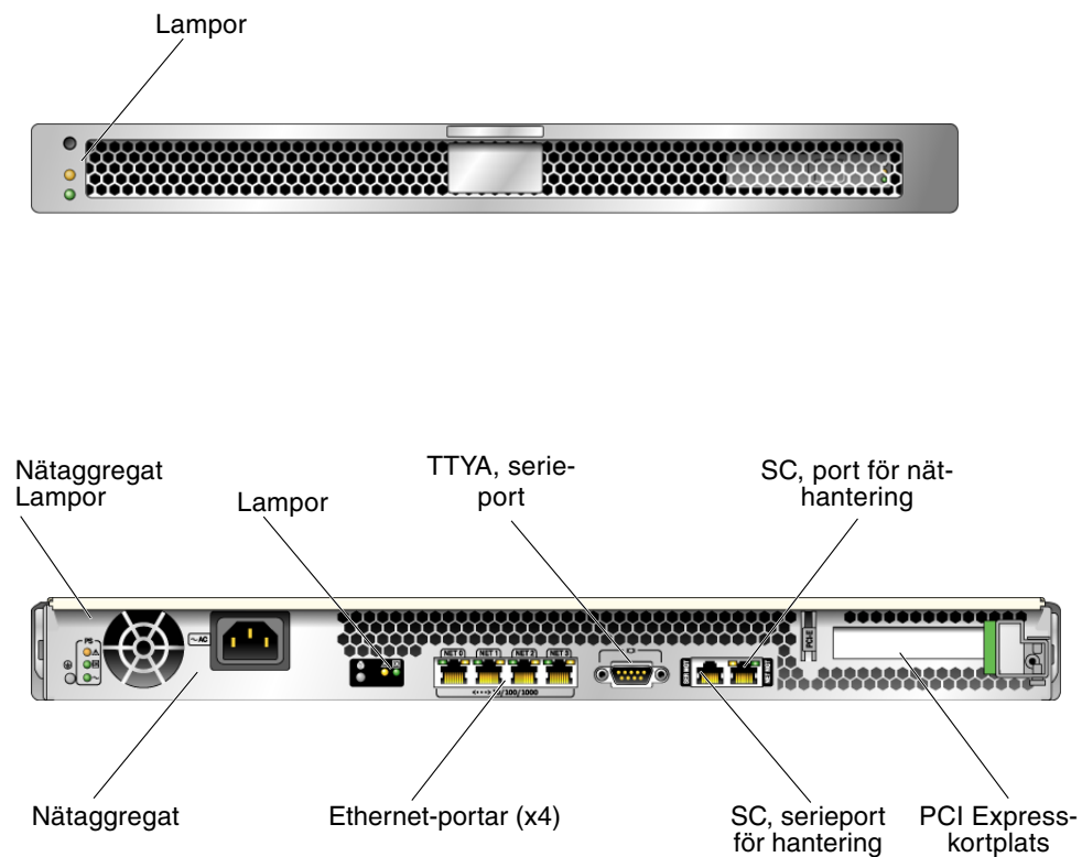
FIGUR 3 Sun SPARC Enterprise T1000, fram- och baksida
