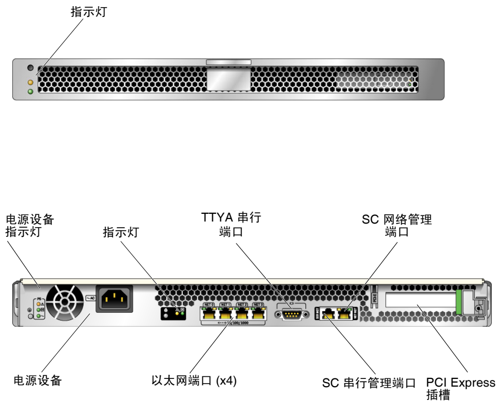
图 3 Sun SPARC Enterprise T1000 服务器的前后面板
