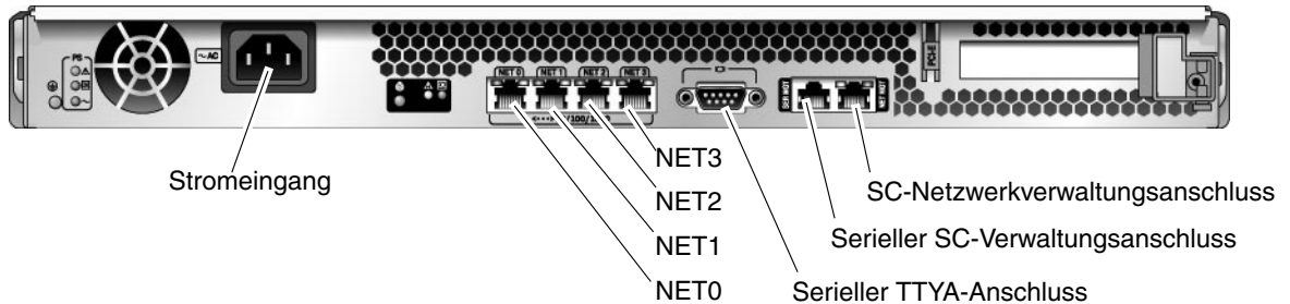
ABBILDUNG 2-9 Anschlüsse auf der Serverrückseite
