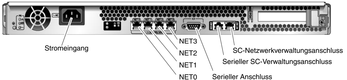
ABBILDUNG 1-5 Position der Anschlüsse auf der Geräterückseite
