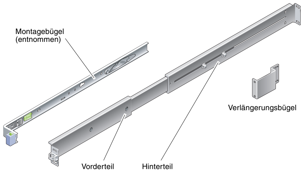
ABBILDUNG 1-2 Schienenbaugruppe
